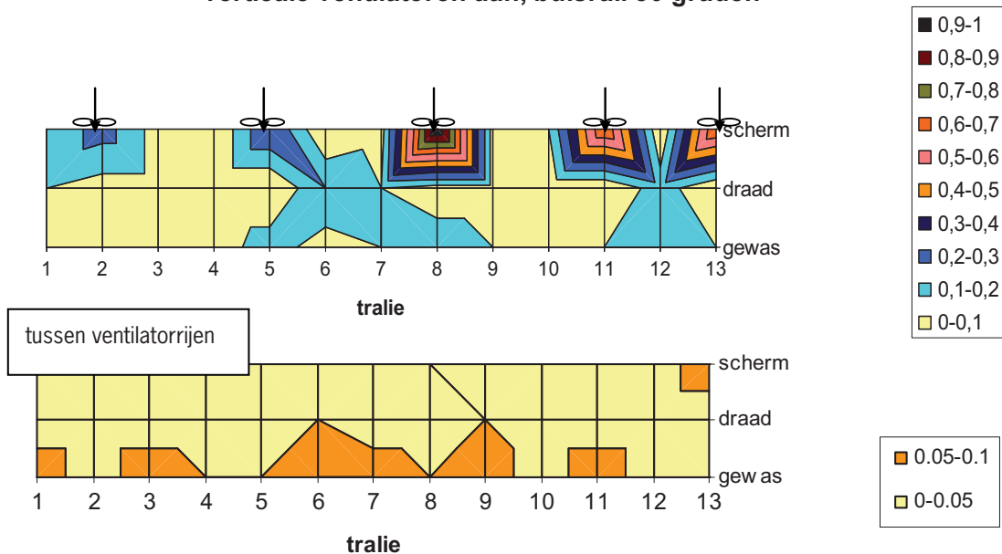
Figuur 27. Luchtsnelheden in m/sec bij gebruik van een Aircobreeze gemeten bij een 1,5 m hoog paprikagewas, op drie hoogten: Net onder het scherm, bij de kop van de plant (draad) en halverwege de plant (gewas).
