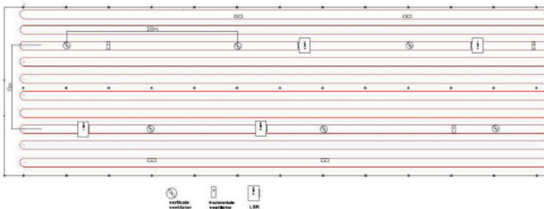
Figuur 15. Plattegrond proefkas met ophangplan ventilatoren.
