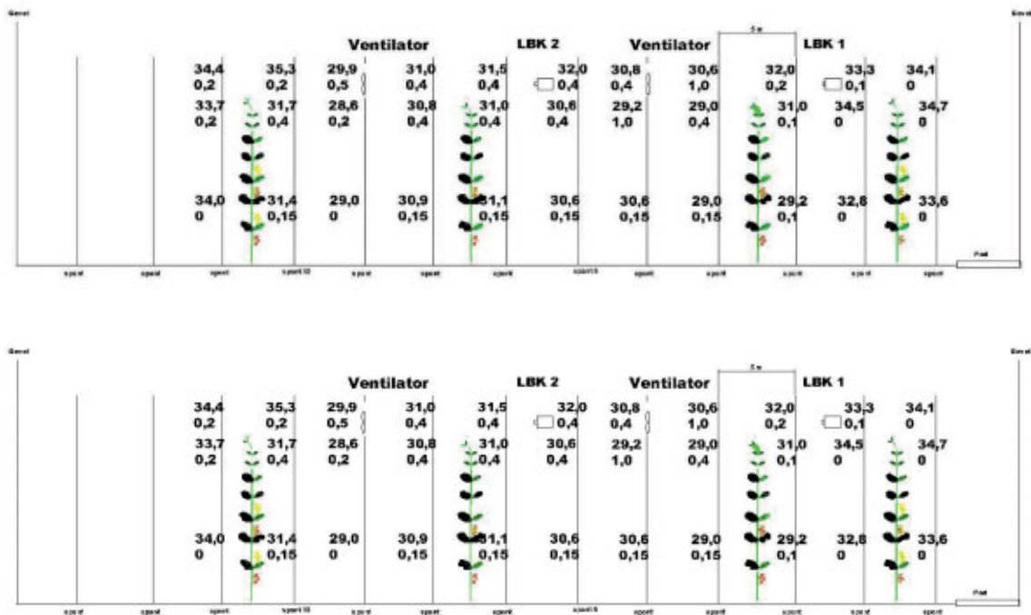
Figuur 8. Zijaanzicht kas: Metingen luchttemperatuur (bovenste getal) en luchtsnelheid in m/sec (onderste getal) in het pad waar de luchtbehandelingskasten hangen. LBK's voorzien van hulpventilatoren op 10 meter afstand. Linker hulpventilator draaide op half vermogen. 940 W/m 2 instraling, verneveling aan. Gevraagd koelvermogen 200 W/m 2 . Ventilator 30 Hz. Raamopening: luwe zijde 45%, windzijde 45%. Datum 12-06-2006, 14.20-15.00 uur.
