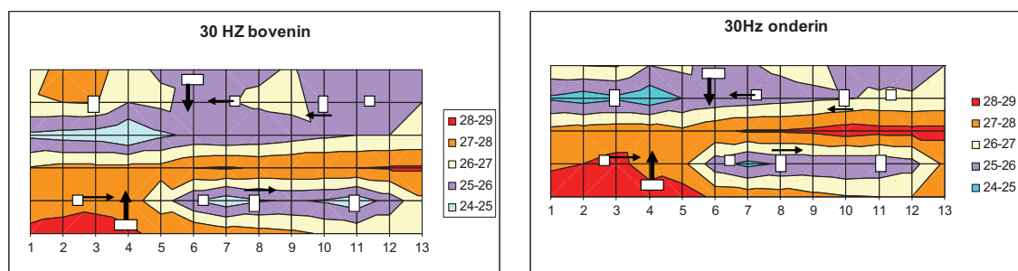
Figuur 13. Horizontaal temperatuurprofiel op twee hoogten. Links op plantkophoogte, rechts op 1m onder de kop. De ventilatoren draaiden op 30Hz vermogen.
