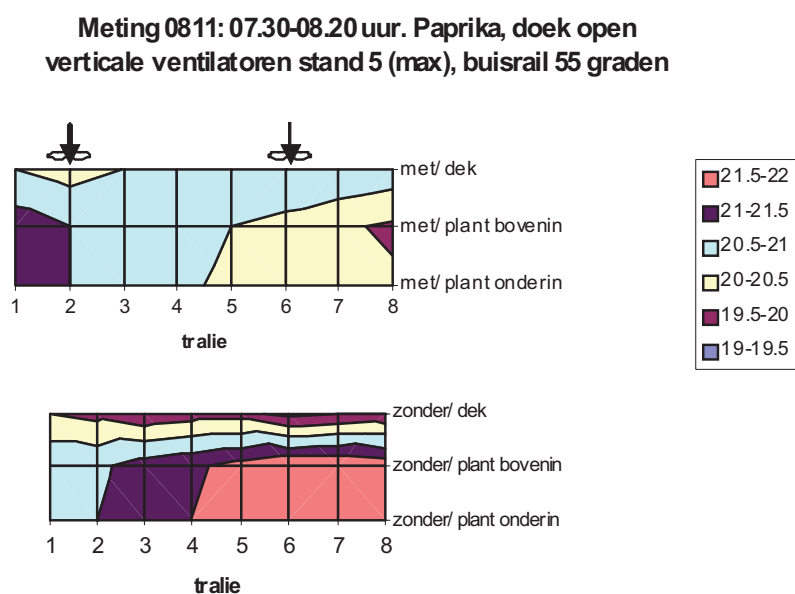
Figuur 23. Verticaal temperatuurprofiel bij paprika bij open schermdoek met en zonder Aircobreeze.
