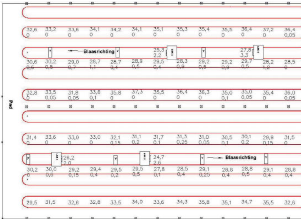
Figuur 10. Plattegrond kas: Luchttemperatuur en luchtsnelheid in m/sec op 1m beneden de koppen van de planten. Alle ventilatoren op maximale stand. Koelvermogen LBK's 120 W/m 2 . Raamstand 55%, verneveling aan. 26-07-2006, 15.00- 16.30 uur.
