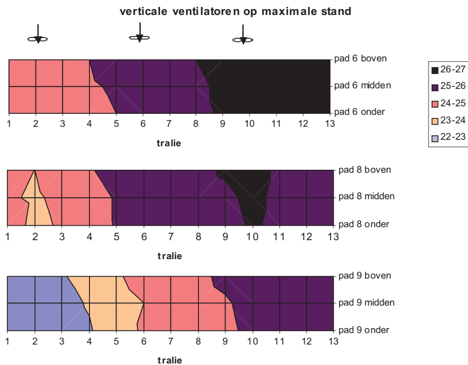
Figuur 19. verticale temperatuurverdeling in 3 paden bij een instraling van 450 \text{ W/m}^2 . Buitentemperatuur 15^\circ\text{C} .
