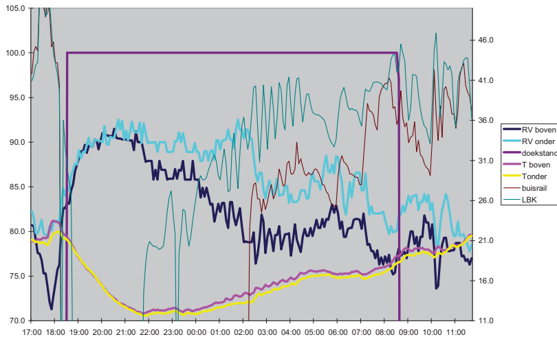
Figuur 4. Verticaal profiel van temperatuur en RV bij gebruik van energiedoek, buisrail en LBK verwarming 26-02-2006.
