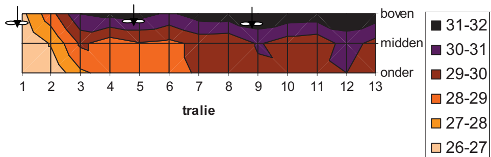
Figuur 18. Verticaal temperatuurprofiel (net boven, halverwege en onderin de plant) over een bedlengte van 13 tralies bij een instraling van 600 \text{ W/m}^2 in het pad onder de Aircobreeze. Buitentemperatuur is 17^\circ\text{C} .
