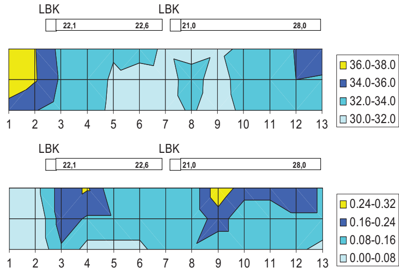
Figuur 6. Zij aanzicht kas: Metingen luchttemperaturen in de verdeelslang achter de luchtbehandelingskasten, de ruimtemtemperatuur en de luchtsnelheden (onderste grafiek) op 3 hoogten. 760 W/m 2 instraling, verneveling aan. Gevraagd koelvermogen 150 W/m 2 . Ventilator 50 Hz. Raamopening: luwe zijde 45%, windzijde 45%. Datum 12-06-2006, 16.00-16.50 uur.
