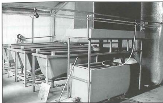
Nederlands recirculatiesysteem, ontwerp Fleuren en Nooyen.
