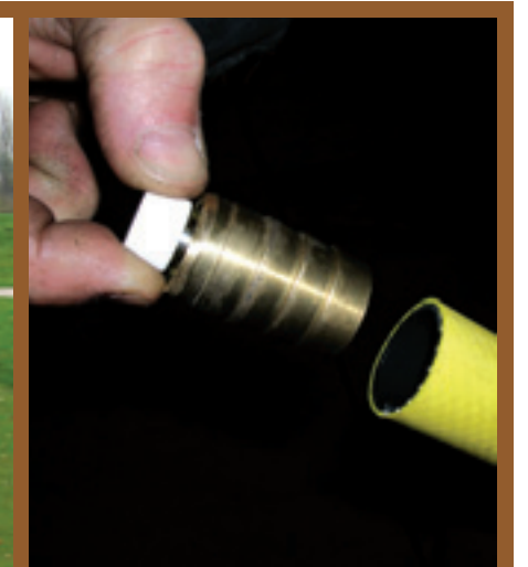
Bij sterk geonduleerde greens geeft een verzwaarde slang een verbeterd resultaat. De slang zal dan beter in de laagtes dauw verwijderen. De drukkoppeling van de beregening sluit zonder druk niet goed af. Een eindstop met ventiel geeft een betere ontluftung bij het vullen van de slang.
