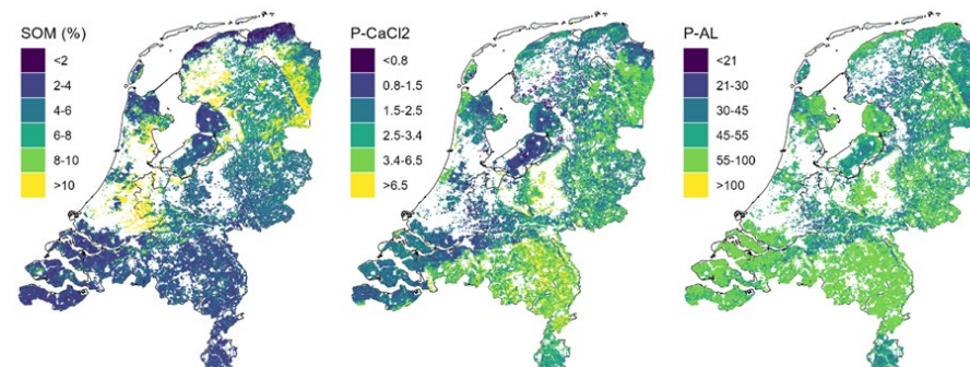
Figuur 2.17 Ruimtelijke variatie in het gehalte aan organische stof (Soil Organic Matter, %), beschikbaar fosfaat voor gewasopname ( P\text{-CaCl}_2 , \text{mg P kg}^{-1} ) en de bodemvoorraad voor fosfaat ( P\text{-AL} , \text{mg P}_2\text{O}_5 100\text{g}^{-1} ) voor bouwlandpercelen in Nederland
