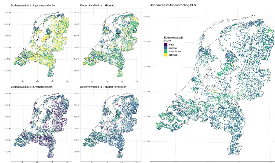
Figuur 2.16 Bodemkwaliteitsbeoordeling van 10.000 willekeurig geselecteerde bouwlandbodems in Nederland in relatie tot de vier ecosysteemdiensten waar de bodem aan bijdraagt. Een blauwe kleur betekent dat er serieuze uitdagingen liggen voor het bodembeheer. Een gele kleur betekent dat het huidige beheer gezorgd heeft voor een optimale bodemkwaliteit
