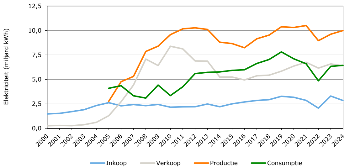
Figuur 4.4 Inkoop, verkoop, productie en gebruik van elektriciteit door de glastuinbouw, 2000-2024 v) v) Cijfers 2024 voorlopig.
