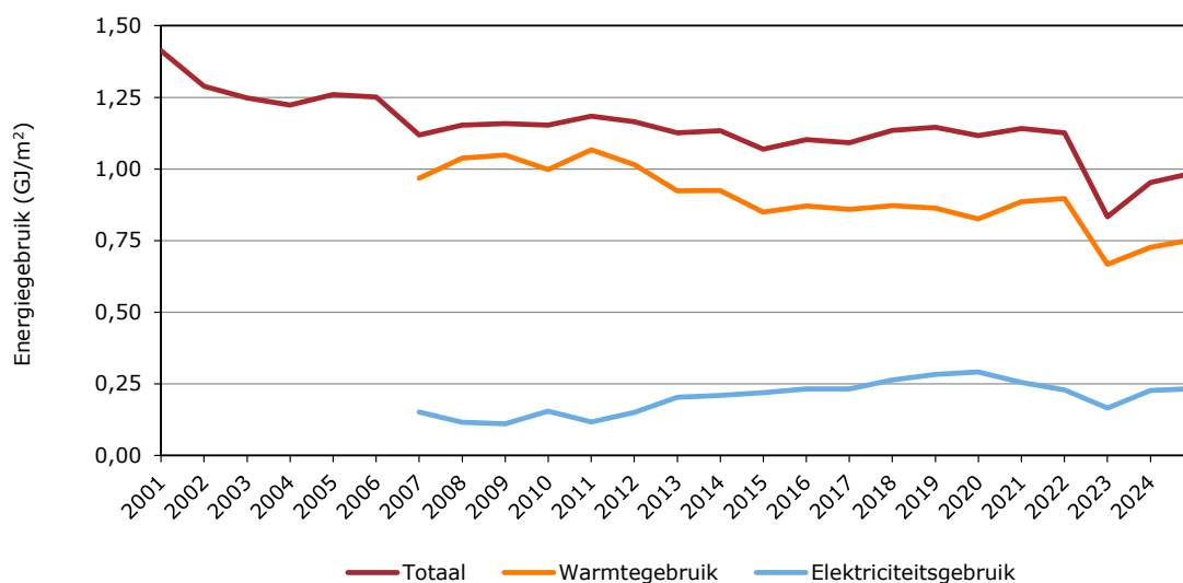
Figuur 2.5 Ontwikkeling gemiddeld energiegebruik glastuinbouw na temperatuurcorrectie, 2000-2024 v) v) Cijfers 2024 voorlopig.
