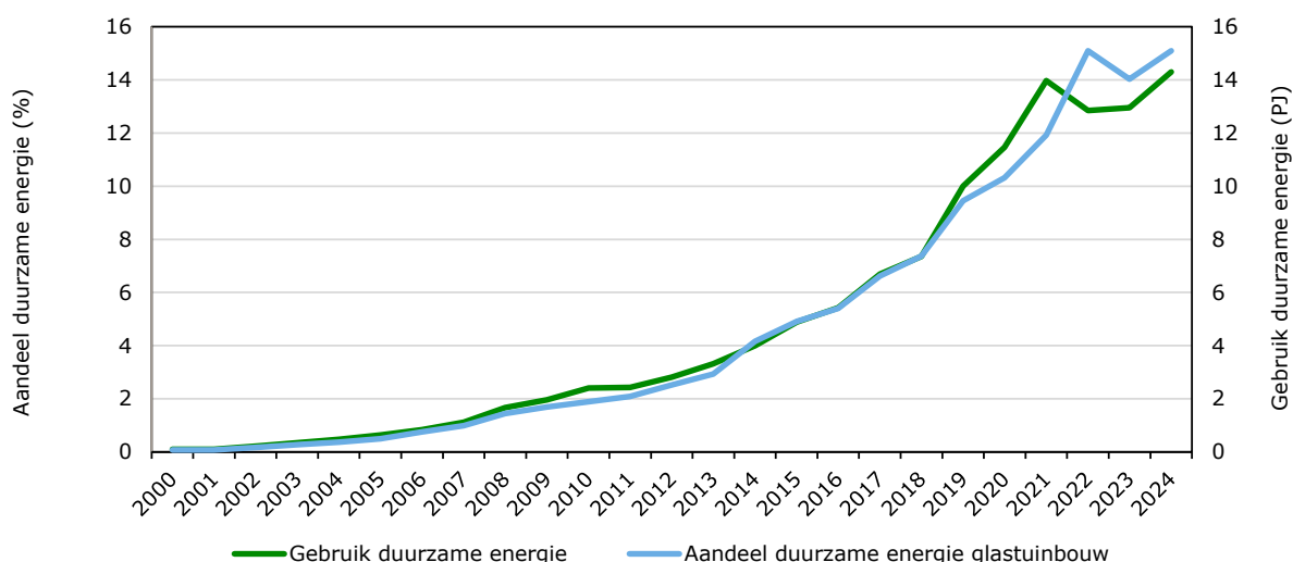
Figuur 3.1 Ontwikkeling gebruik (PJ) en aandeel (%) duurzame energie in de glastuinbouw, 2000-2024 v) v) Cijfers 2024 voorlopig.
