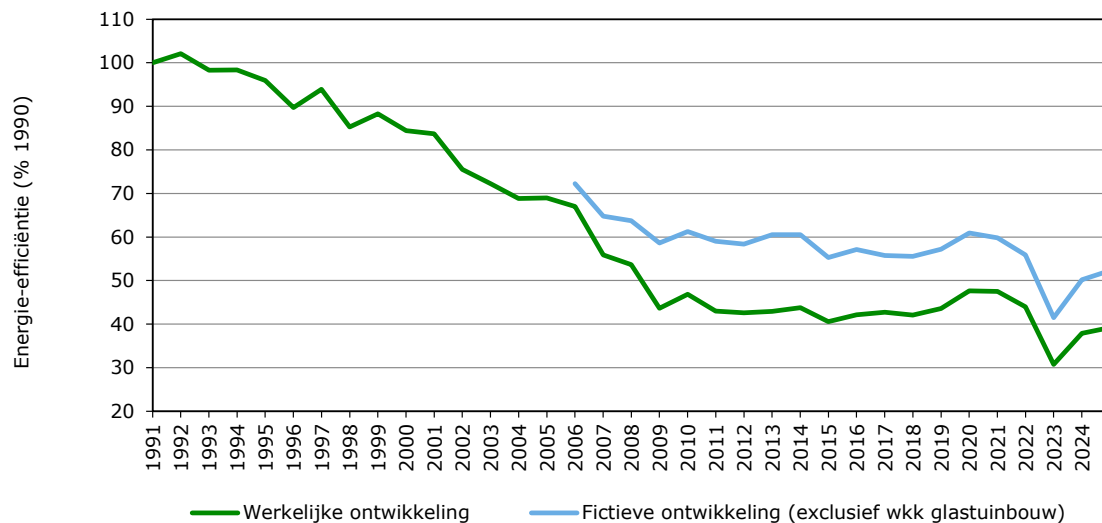
Figuur 2.6 Energie-efficiëntie productieglastuinbouw per jaar met en zonder wkk glastuinbouw, 1990-2024 v) v) Cijfers 2024 voorlopig.
