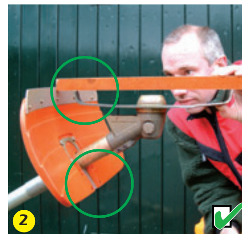
2 Speciale shredderkap: Voldoende overlap met maaivlak en voldoende bescherming aan de bovenkant. Voldoet aan de CE-markering.
