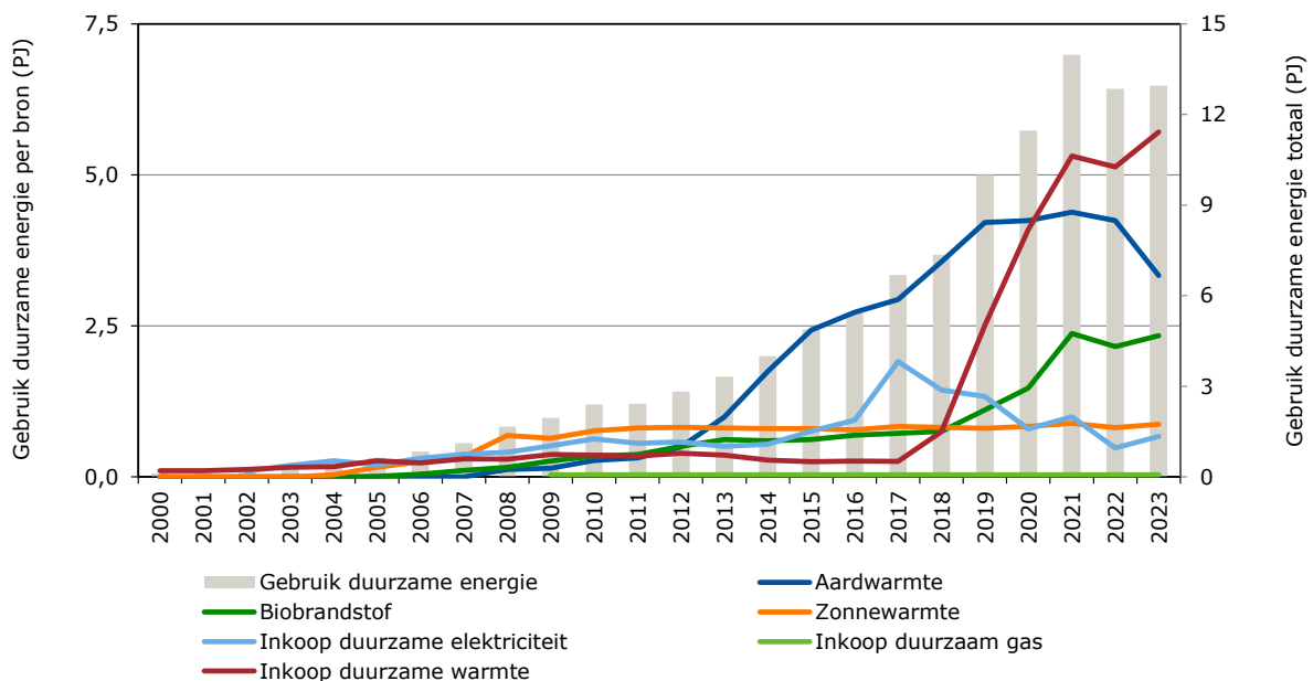
Figuur 3.2 Ontwikkeling gebruik duurzame energie in de glastuinbouw per bron en totaal 2000-2023 v) v) Cijfers 2023 voorlopig.
