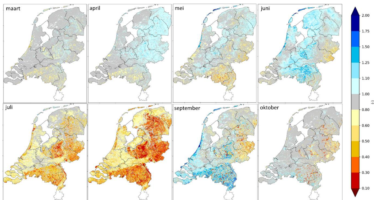
Figuur 2.4 Berekende relatieve bodemvochtgehalten in de bovenste 10 cm van de bodem voor de maanden maart t/m oktober van 2022. Hierbij is het bodemvochtgehalte van 2022 gedeeld door het langjarig gemiddelde bodemvochtgehalte over de periode 1990-2017. Blauwe kleuren tonen relatief hogere bodemvochtgehalten in 2022 ten opzichte van het gemiddelde en geel/rode kleuren tonen relatief lagere bodemvochtgehalten in 2022.
