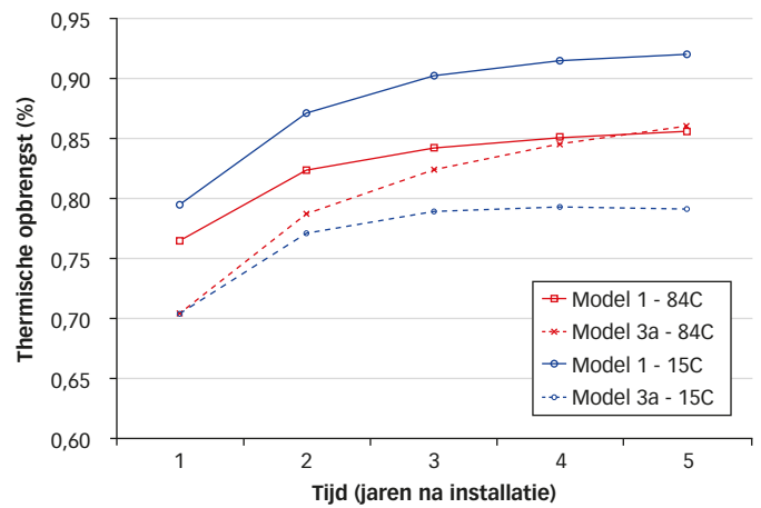
AFBEELDING 2: GEMODELLEERD THERMISCH RENDEMENT GEDURENDE DE EERSTE 5 JAAR VAN DE WARMTE PUT BIJ EEN WARMTE-OPSLAG INSTALLATIE MET INJECTIETEMPÉRATUUR VAN 15°C EN 84°C VOOR UNIFORME (MODEL 1) EN HETEROGENE (MODEL 3A) WATERVOEREND PAKKETTEN (AFKOMSTIG VAN PINEAUD, 2014).
