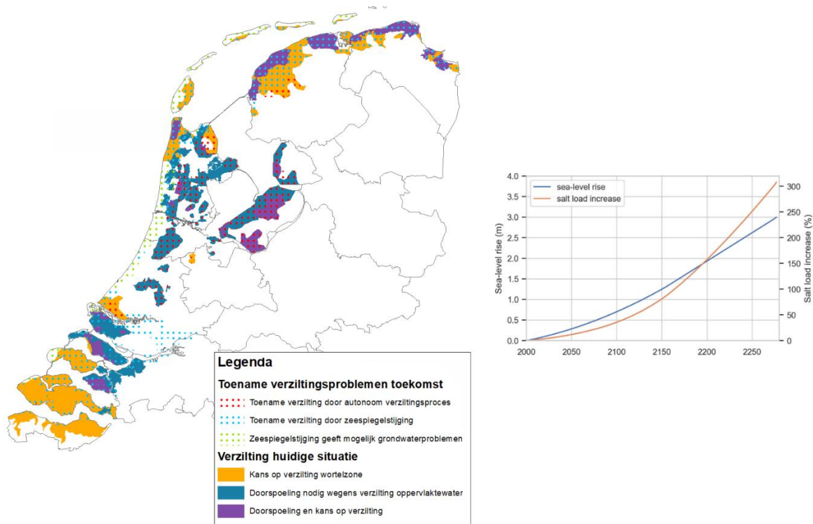
Afbeelding 7 a. De verziltingsrisicokaart geeft aan de hand van modelberekeningen een landelijk beeld van het risico op verzilting, bij 1 meter zeespiegelstijging in het jaar 2100 (Delsman, 2021). De kaart is met name gericht op landbouw en waterbeheer; diepere verziltingsproblemen verder landinwaarts maken geen deel uit van deze kaart, zoals bijvoorbeeld het verzilten van diepe winputten. b. in het kustgebied zal de toename van de zoutbelasting door zeespiegelstijging (t.o.v. de huidige situatie, in %) plaatsvinden (Delsman et al., 2022). De grootste verandering in zoetwatervraag vindt plaats met name de polders van Noord-Holland, Friesland en Groningen.
