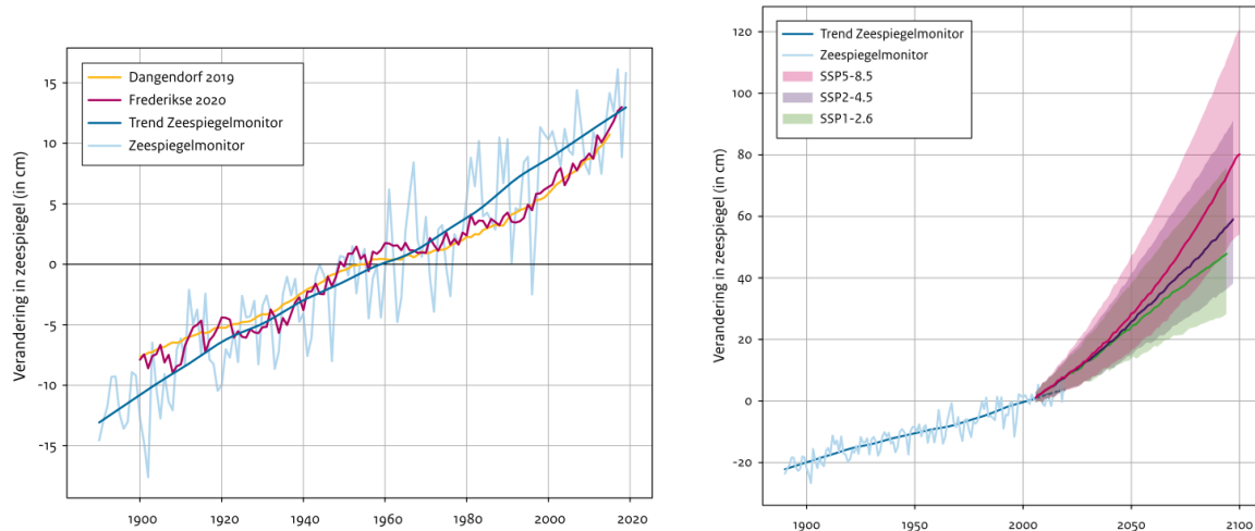
Afbeelding 4 Links: Zeespiegelstijging voor de Nederlandse kust (blauw gebaseerd op zes getijddestations) versus twee reconstructies van de wereldgemiddelde zeespiegelstijging ( KNMI, 2021 ); Rechts: Zeespiegel aan de Nederlandse kust zoals waargenomen en volgens de nieuwe, indicatieve zeespiegelprojecties. De getrokken lijnen in groen, paars, rood geven de mediaan aan van die projecties, het gekleurde gebied de 90%-bandbreedte ( KNMI, 2021 ). SSP staat voor Shared Socioeconomic Pathway en beschrijft verschillende emissiescenario's (gelieerd aan de onderliggende socio-economische ontwikkelingen) waarbij de wereldwijde temperatuurstijging tegen het einde van de 21 ste eeuw beperkt blijft tot gemiddeld 1.8, 2.7 en 4.4 graden Celsius boven pre-industriële niveaus voor SSP2.6, SSP4.5 en SSP8.5, respectievelijk. Zie webportal Dutch Sea Level Change .
