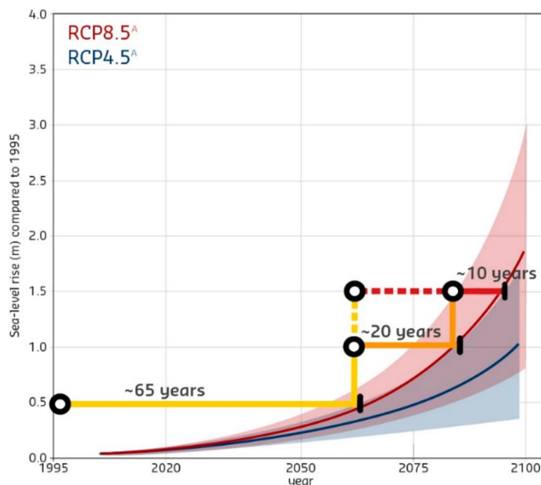
Afbeelding 10 Het effect van versnelde zeespiegelstijging op de levensduur van investeringen. In de huidige situatie houdt een ontwerp voor 50 cm 65 jaar aan. De mogelijke versnelling later deze eeuw verkort de levensduur van een ontwerp van 50 cm tot ongeveer 10 jaar ( Haasnoot et al., 2020 ; Van Alphen et al., 2022 ).
