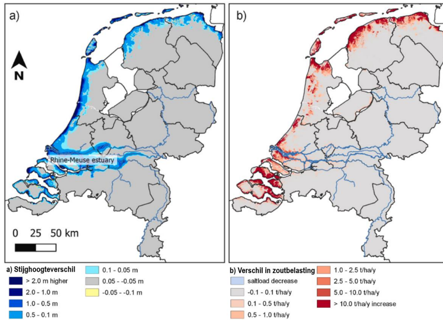
Afbeelding 6 a. De invloedssfeer van een zeespiegelstijging in het grondwatersysteem. Modelberekeningen laten bij een scenario van 3m zeespiegelstijging (jaar 2277) het stijghoogte verschil (in m) zien in de eerste watervoerende laag ten opzichte van het scenario zonder zeespiegelstijging, b. verschil in zoutbelasting (in ton Cl-/ha/j) bij een 3m zeespiegelstijging (jaar 2277). De zoutbelasting wordt gedefinieerd als de opwaartse stroming van chloride van de eerste watervoerende laag naar de bovenste opsluitende eenheid (Delsman et al., 2022, Delsman et al., 2023).
