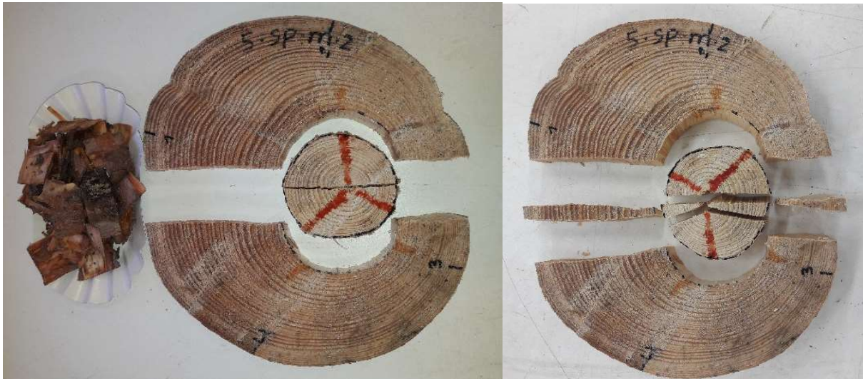
Figuur 2.5 Scheiding van de bast, spinthout en kernhout (links) en de extractie van spint- en kernhoutstukken voor de conversie van versgewicht naar drooggewicht en de dichtheidsmetingen.
