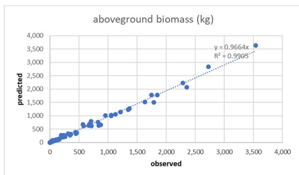
Figuur 2.4 Verhouding tussen geschat en gemeten stam biomassa (links) en geschat en gemeten bovengronds biomassa van Beuk.
