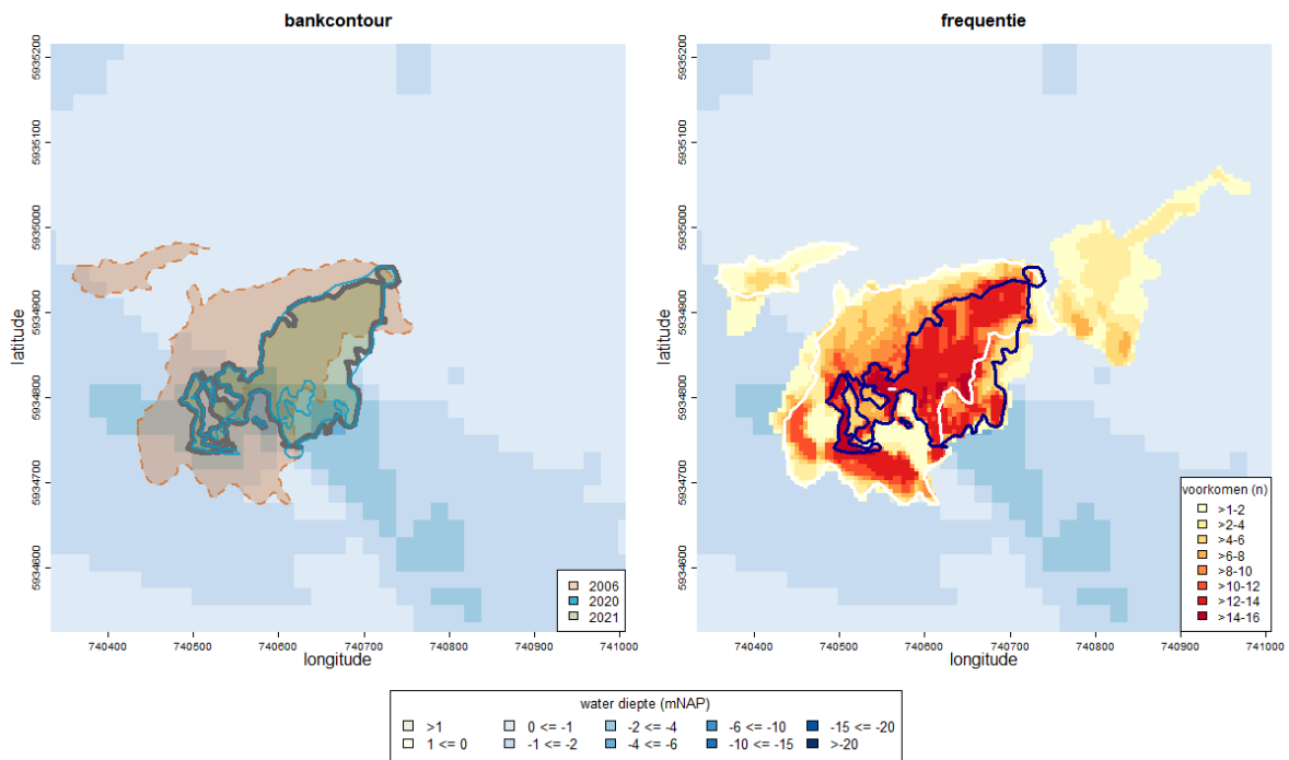
Figuur 3.8 Contouren van de mosselbank 736 (onder Rottumeroog) voor verschillende jaren. In de linker figuur worden de contouren weergegeven zoals bepaald werd in de eerste meting (in 2006 en lichtbruin ingekleurd), zoals bepaald werd in 2021 (lichtgroen ingekleurd) en zoals bepaald werd in 2020 (lichtblauw omlijnd). In de rechterfiguur wordt op een raster van 5 bij 5 m weergegeven hoe vaak de rastercellen zich binnen de mosselbank bevonden (hoe roder, hoe frequenter) voor de jaren dat de bank bezocht werd en er een contour beschikbaar was. In deze figuur wordt met een witte lijn de contour van de eerste meting weergegeven en met een donkerblauw doorgetrokken lijn de contour van de bank in 2020. De waterdiepte is weergegeven op een raster en betreft gegevens die ingewonnen zijn in de periode 2013 tot en met 2019.
