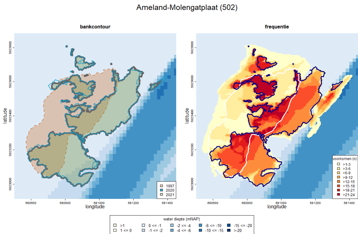
Figuur 3.1 Contouren van de mosselbank 502 (onder Ameland) voor verschillende jaren. In de linker figuur worden de contouren weergegeven zoals bepaald werd in de eerste meting (in 1997 en lichtbruin ingekleurd), zoals bepaald werd in 2021 (lichtgroen ingekleurd) en zoals bepaald werd in 2020 (lichtblauw omljnd). In de rechterfiguur wordt op een raster van 5 bij 5 m weergegeven hoe vaak de rastercellen zich binnen de mosselbank bevonden (hoe roder, hoe frequenter) voor de jaren dat de bank bezocht werd en er een contour beschikbaar was. In dit figuur wordt met een witte lijn de contour van de eerste meting weergegeven en met een donkerblauw doorgetrokken lijn de contour van de bank in 2021. De waterdiepte is weergegeven op een raster en betreft gegevens die ingewonnen zijn in de periode 2013 tot en met 2019.
