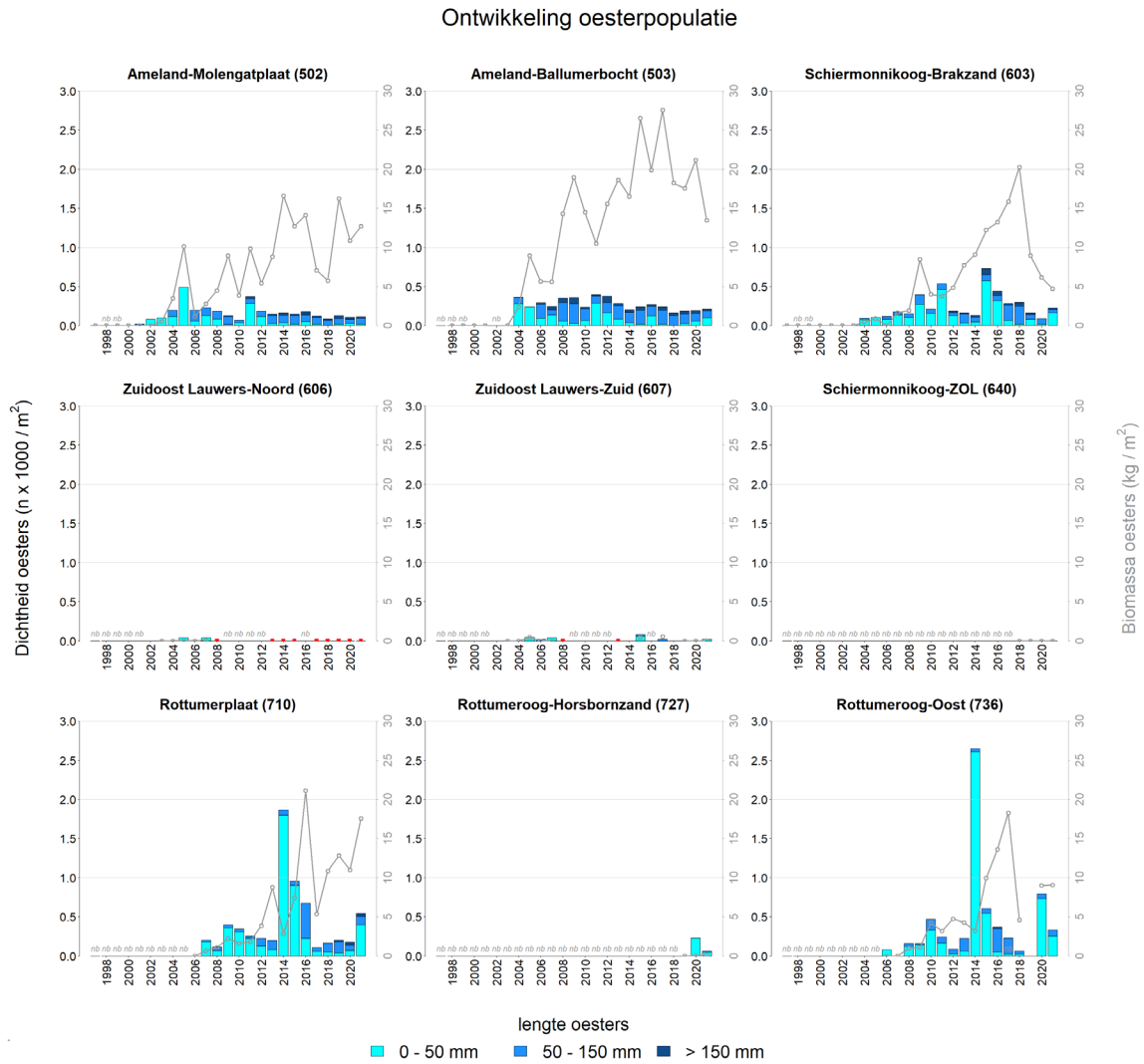
Figuur B5.1 Ontwikkeling van jaargemiddelde dichtheid (n x 1000/m 2 ) en biomassa (kg natgewicht/m 2 ) Japanse oesters zoals aangetroffen in de vierkantmonsters (1/20 m 2 ) voor de banken 502, 503, 603, 606, 607, 640, 710, 727 en 736 in de periode 1997 t/m 2021 (of tot wanneer ze bezocht zijn/aanwezig waren). De dichtheden (onderverdeeld in drie lengteklassen) zijn weergegeven met balken en uitgezet op de linker y-as. De oesterbiomassa's zijn met grijze lijnen weergegeven en uitgezet op de rechter y-as. Wanneer een bank wel bezocht werd maar niet aanwezig was, is dit met een rode stip aangegeven.
