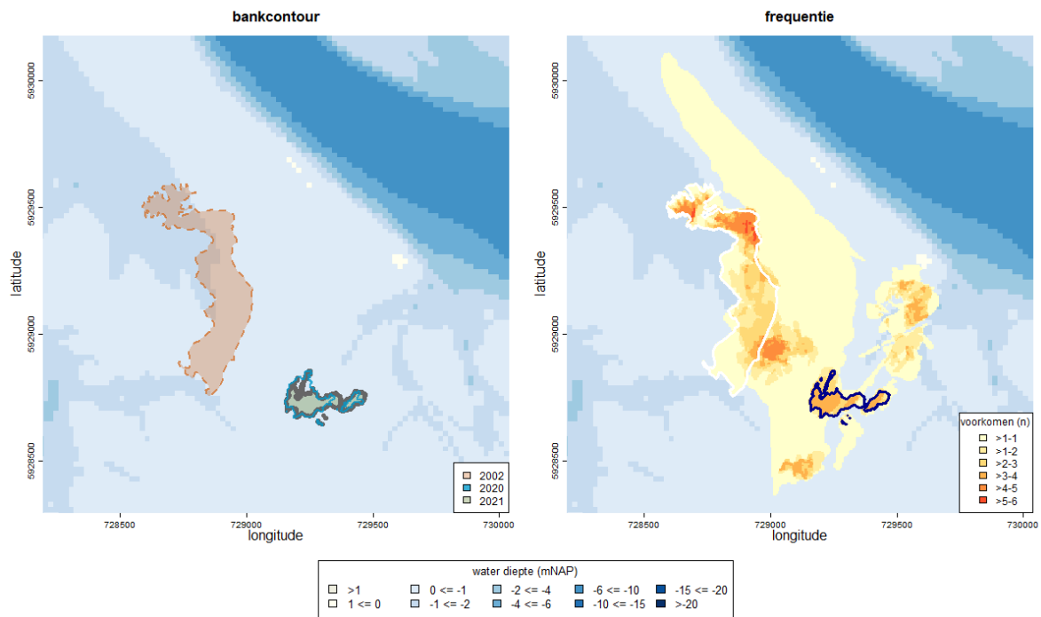
Figuur 3.4 Contouren van de mosselbank 607 (onder Rottumerplaat) voor verschillende jaren. In de linker figuur worden de contouren weergegeven zoals bepaald werd in de eerste meting (in 2002 en lichtbruin ingekleurd), zoals bepaald werd in 2021 (lichtgroen ingekleurd) en zoals bepaald werd in 2020 (lichtblauw omlijnd). In de rechterfiguur wordt op een raster van 5 bij 5 m weergegeven hoe vaak de rastercellen zich binnen de mosselbank bevonden (hoe roder, hoe frequenter) voor de jaren dat de bank bezocht werd en er een contour beschikbaar was. In dit figuur wordt met een witte lijn de contour van de eerste meting weergegeven en met een donkerblauw doorgetrokken lijn de contour van de bank in 2021. De waterdiepte is weergegeven op een raster en betreft gegevens die ingewonnen zijn in de periode 2013 tot en met 2019.
