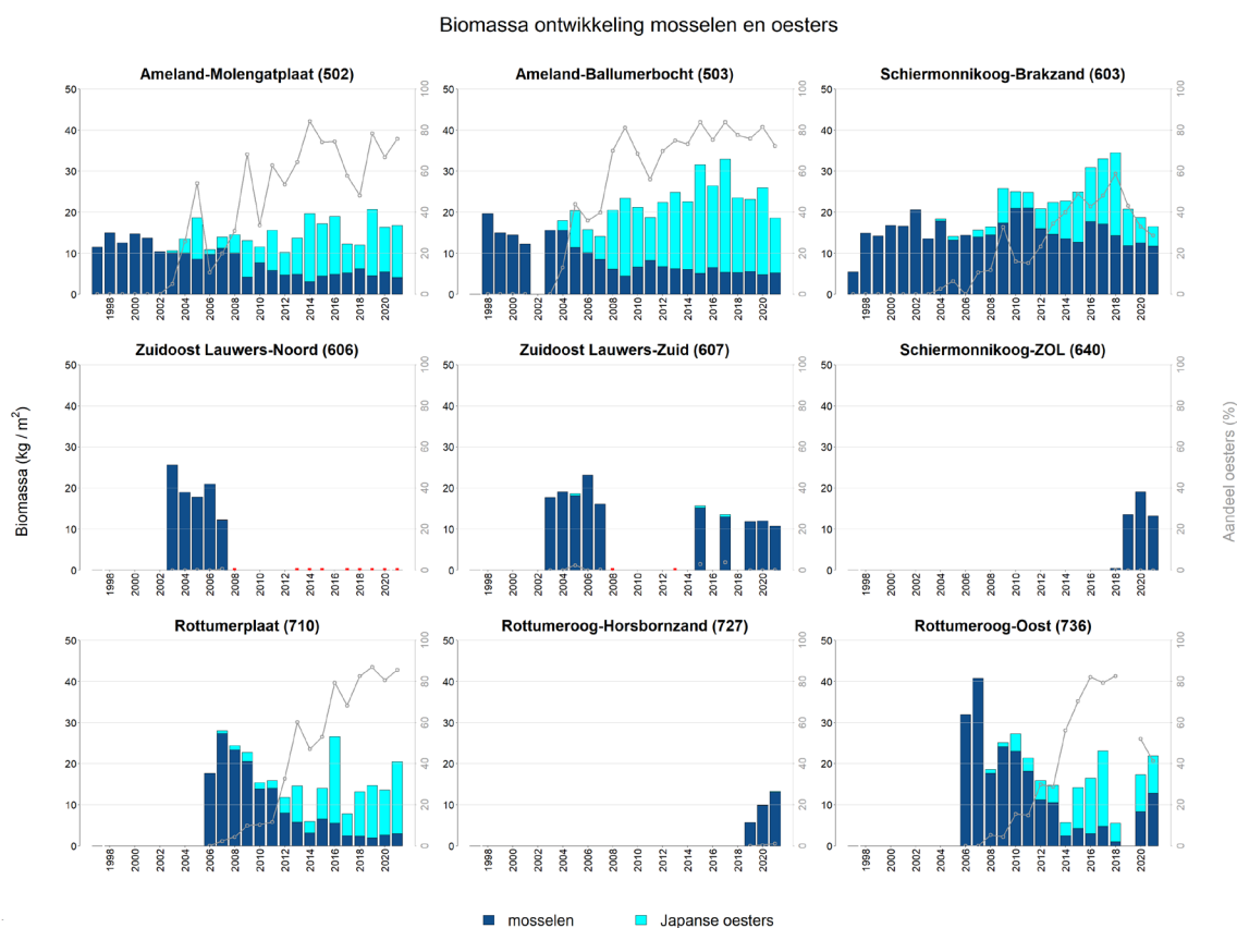
Figuur 3.12 Ontwikkeling van de jaargemiddelde biomassa mosselen en Japanse oesters (uitgedrukt in kg natgewicht/m 2 en weergegeven in staven ten opzichte van de linker y-as) en het aandeel oesters (uitgedrukt in procenten en weergegeven in lijndiagram ten opzichte van de rechter y-as) in de mossel-/oesterbiomassa zoals aangetroffen in de vierkantmonsters (0,05 m 2 ) voor de banken 502, 503, 603, 606, 607, 640, 703, 710, 727 en 736 in de periode 1997 t/m 2021 (of tot wanneer ze bezocht zijn/aanwezig waren). Wanneer een bank wel bezocht werd, maar niet aanwezig was, is dit met een rode stip aangegeven.
