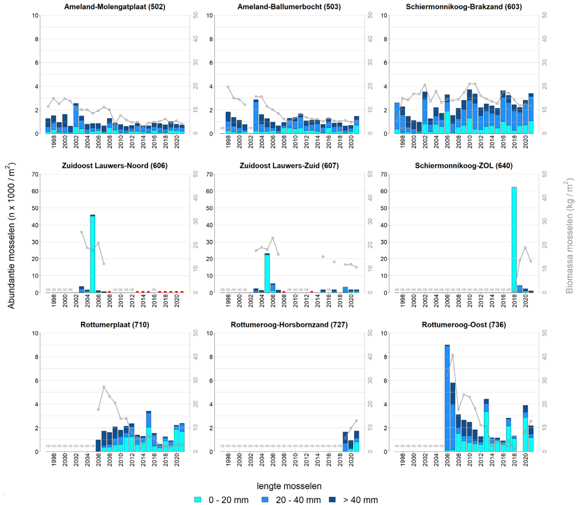
Figuur B4.1 Ontwikkeling van jaargemiddelde dichtheid ( n \times 1000/m^2 ) en biomassa ( kg \text{ natgewicht}/m^2 ) mosselen zoals aangetroffen in de vierkantmonsters ( 0,05 m^2 ) voor de banken 502, 503, 603, 606, 607, 640, 710, 727 en 736 in de periode 1997 t/m 2021 (of tot wanneer ze bezocht zijn/aanwezig waren). De dichtheden (onderverdeeld in drie lengteklassen) zijn weergegeven met balken en uitgezet op de linker y-as. De mosselbiomassa's zijn met grijze lijnen weergegeven en uitgezet op de rechter y-as. Wanneer een bank wel bezocht werd maar niet aanwezig was, is dit met een rode stip aangegeven.
