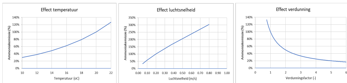
Figuur 12 Modelmatige relaties tussen de relatieve ammoniakemissie enerzijds en anderzijds respectievelijk de temperatuur van het emitterende oppervlak (20°C = 100%), luchtsnelheid boven het emitterend oppervlak (0,20 m/s = 100%) en verdunningsfactor van de mest (1 = 100%; 1 betekent geen verduunning) [2]. Deze relaties zijn gebruikt voor bepaling van de ammoniakemissie per m 2 emitterend oppervlak in biologische stallen in Tabel 5.
