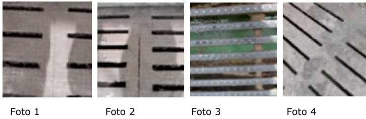
Figuur 3 Foto's van de verschillende typen roostervloeren in het onderzoek van Aarnink et al. [10]. Foto 1 = composietrooster 8 cm brede balk; Foto 2 = composietrooster 4 cm brede balk; Foto 3 = metalen driekantrooster met profiel 1 cm brede balk; Foto 4 = betonrooster 8 cm brede balk.
