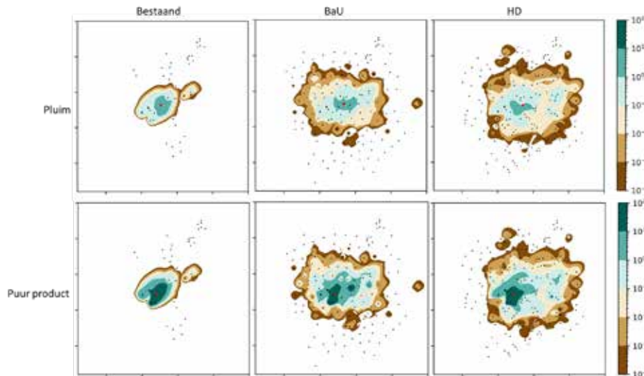
Afbeelding 1. De verspreiding van de verontreiniging na 10 jaar voor de bestaande (links), de BaU- (midden) en HD- (rechts) scenario's voor de pluimverontreiniging (boven) en de verontreiniging met puur product (onder). Elke subplot toont de concentratie in een gebied van 3x3 kilometer. Elke zwarte stip is een OBES-put, en de rode stip geeft het massamiddelpunt van de pluim.
