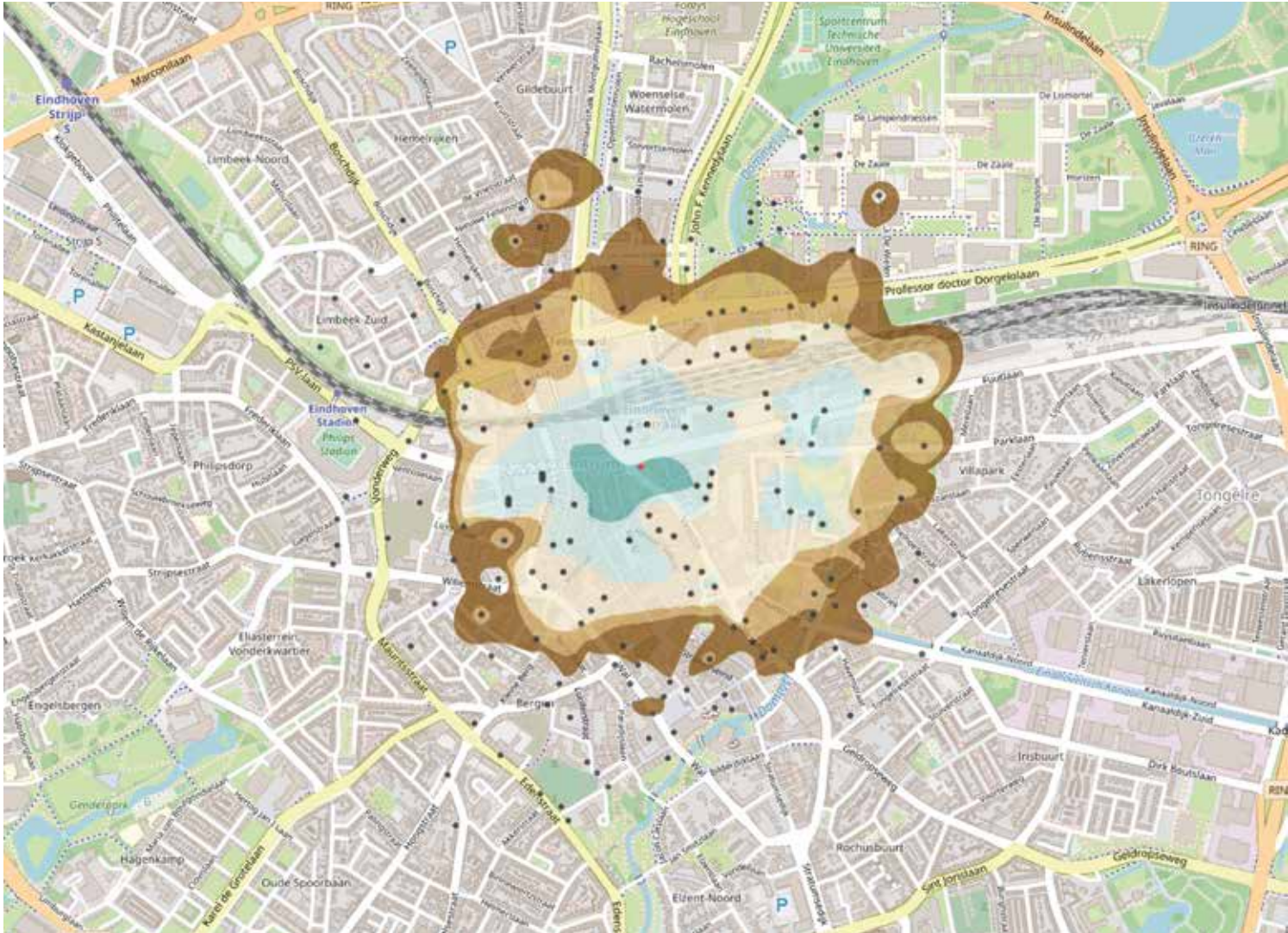
Binnenstad Eindhoven: gesimuleerde verspreiding van een fictieve verontreiniging door bestaande en geplande open bodemenergiesystemen en achtergrondstroming
