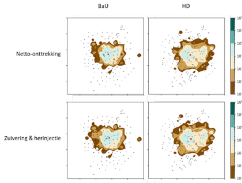
Afbeelding 2. Het effect van verschillende beheersmaatregelen op de verspreiding van een verontreinigingspluim voor de twee toekomstscenario's, BaU (links) en HD (rechts). Elke subplot toont de concentratie van de verontreiniging in een gebied van 3x3 kilometer, de contouren geven het verdunningsniveau van de verontreiniging aan. Elke zwarte stip is een OBES-bron, en de rode stip geeft het massamiddelpunt van de pluim aan.
