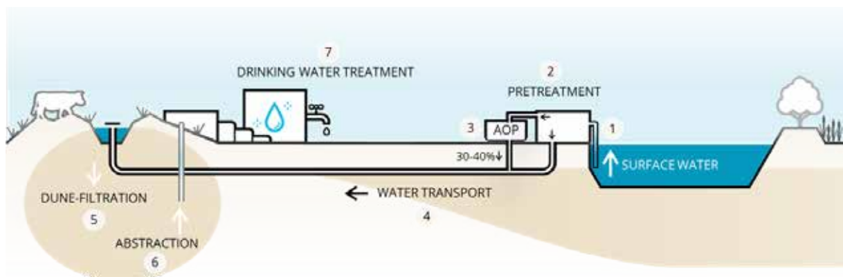
Afbeelding 1. Schema van de drinkwaterzuivering door Dunea. Oppervlaktewater wordt ingenomen (1) en voorbehandeld met snelle zandfiltratie (2) en daarna deels (30-40%) met geavanceerde oxidatie (3). Dit voorbehandelde water wordt getransporteerd naar het duininfiltratiesysteem (4) en gefiltreerd (5), waarna water wordt onttrokken (6) voor drinkwaterproductie (7).
