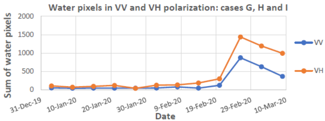
Figuur 3.4: Boven: detailbeeld van de MNSWI (Modification of Normalized Difference Water Index) op 3 maart 2020 voor percelen G, H en I. Onder: het verloop van de omvang van de plasvorming op percelen G, H en I op basis van SAR (VH en VV zijn verschillende polarisaties van de radarbeelden).
