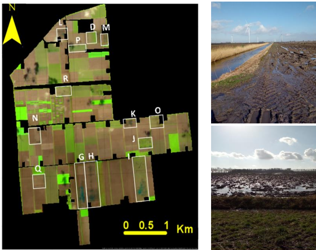
Figuur 3.3: Voorbeelden van detectie van plassen op het land in maart 2020 in de Vuursteentocht, satellietbeeld van 16 maart 2020 (bruin is onbedekt, groen is bedekt, blauw/turquoise is plasvorming, witte kaders geven blijvende plassen van november 2019 tot maart 2020 aan). Rechts veldfoto's van 3 maart 2020.
