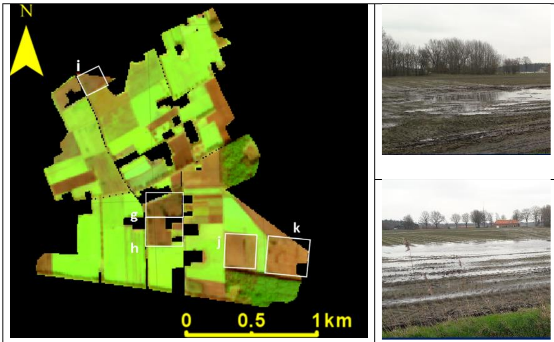
Figuur 3.5: Voorbeelden van detectie van plassen op het land in maart 2020 in de Vinkenloop satellietbeeld van 18 maart 2020 (bruin is onbedekt, groen is bedekt, blauw/turquoise is plasvorming, witte kaders geven blijvende plassen van november 2019 tot maart 2020 aan). Rechts veldfoto's van 5 maart 2020.
