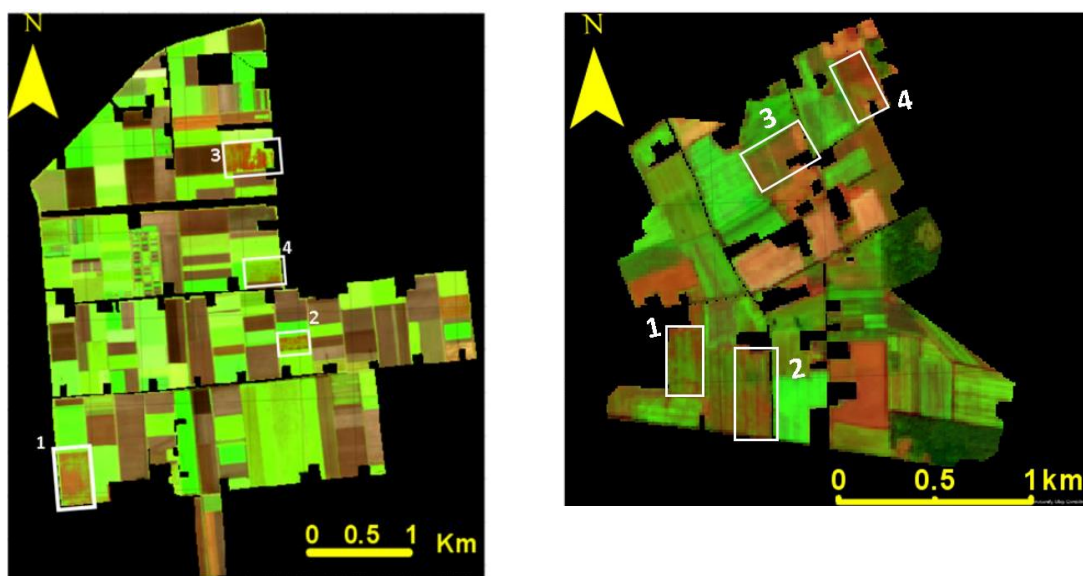
Figuur 3.2: Voorbeelden van detectie van plekken binnen bedekte percelen die minimaal 1 maand kaal bleven, 4 gevallen per gebied (links Vuursteentocht 30 okt 2019, rechts Vinkenloop 6 aug 2018). Bruin is onbedekt, groen is bedekt.
