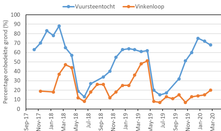
Figuur 3.1: Percentage onbedekte percelen in de Vuursteentocht en de Vinkenloop
