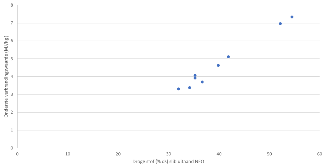
FIGUUR 4.8 RELATIE DROGESTOF EN ONDERSTE VERBRANDINGSWAARDE SLIB (MJ/KG)
