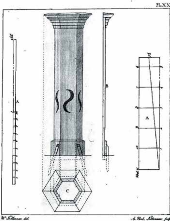
< 'Bouwtekening' van een boomkoker uit Beginselen van het bouwkunstig teekenen (1829).
