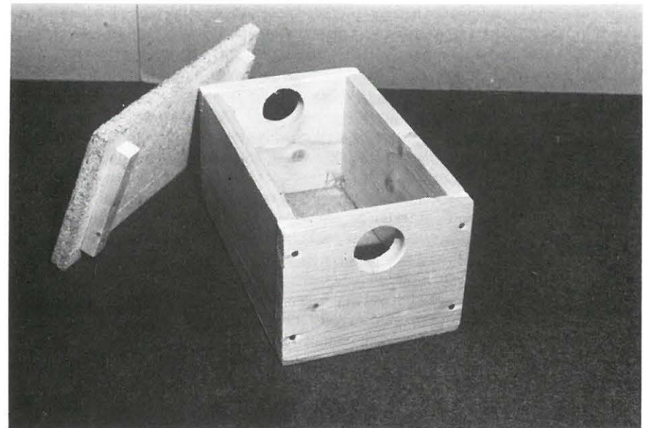
Muizenvoerkist met openingen aan korte kant i.v.m. plaatsing indien nodig op balken.
