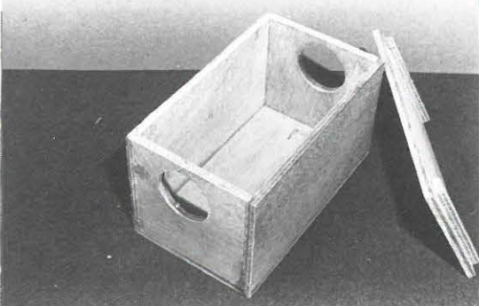
"voerkist voor de bestrijding van bruine en zwarte ratten in gebouwen"
