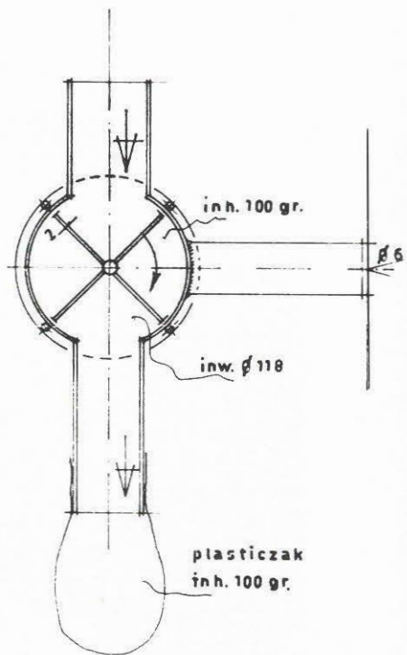
DOORSNEDE
