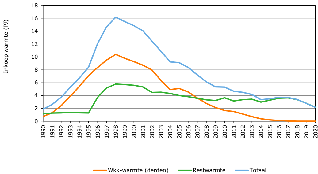
Figuur 4.5 Inkoop van niet-duurzame warmte door de glastuinbouw v) v) Cijfers 2020 voorlopig.
