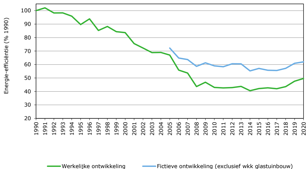
Figuur 2.3 Energie-efficiëntie van de productieglastuinbouw per jaar met en zonder wkk glastuinbouw v)
