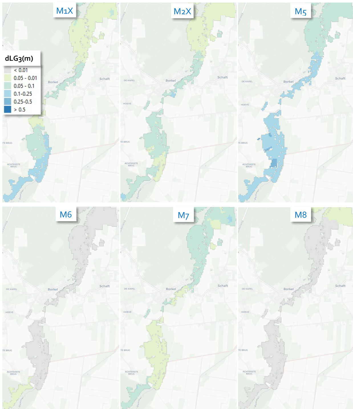
Figuur 82. Met het LHM gesimuleerde stijging van de laagste grondwaterstand (dLG3) onder de grondwaterafhankelijke natuur van de Dommel en omgeving door een aantal hypothetische maatregelen: M1X – Drinkwaterwinning stoppen, M2X – Beregening stoppen, M5 – Stuwpeil en drainageniveau +30 cm; M6 – Ondergrondse zoetwaterberging, M7 – Naaldbos naar heide, M8 – Afkoppelen bebouwd gebied.
