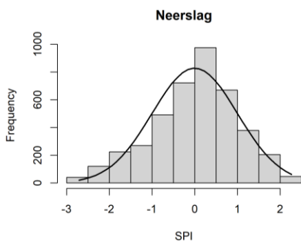
Figuur 100. Voorbeeld van de verdeling van SPI-waarden gebaseerd op neerslagdata gefit met een Gammaverdeling en omgezet naar de standaardnormale verdeling.
