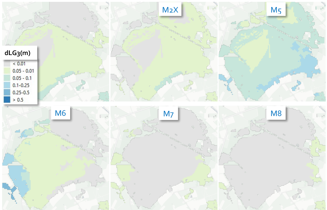
Figuur 8o. Met het LHM gesimuleerde stijging van de laagste grondwaterstand ( dLG_3 ) onder de grondwaterafhankelijke natuur van Het Korenburger veen en omgeving door een aantal hypothetische maatregelen: M_{1X} – Drinkwaterwinning stoppen, M_{2X} – Beregening stoppen, M_5 – Stuwpeil en drainageniveau +30 cm; M_6 – Ondergrondse zoetwaterberging, M_7 – Naaldbos naar heide, M_8 – Afkoppelen bebouwd gebied.
