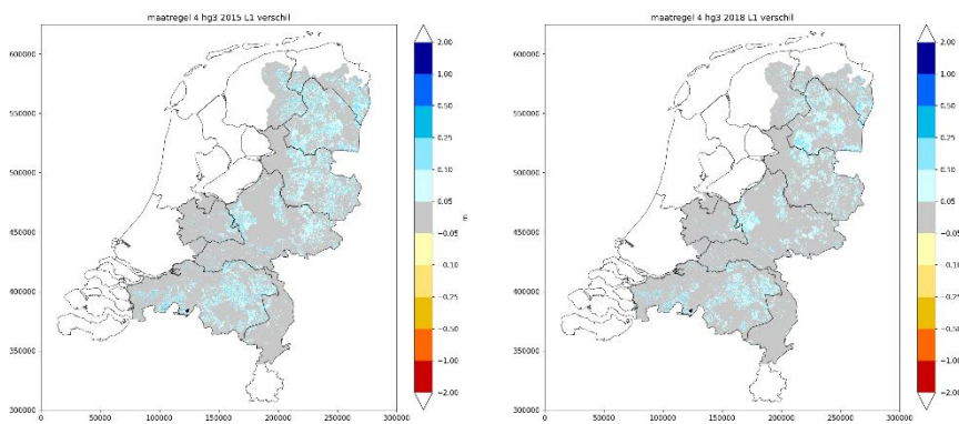
Figuur 31. Het berekende effect van een slootbodempluiging van het tertiair ontwateringsstelsel van 30 cm op de HG 3 voor 2015 en 2018.
