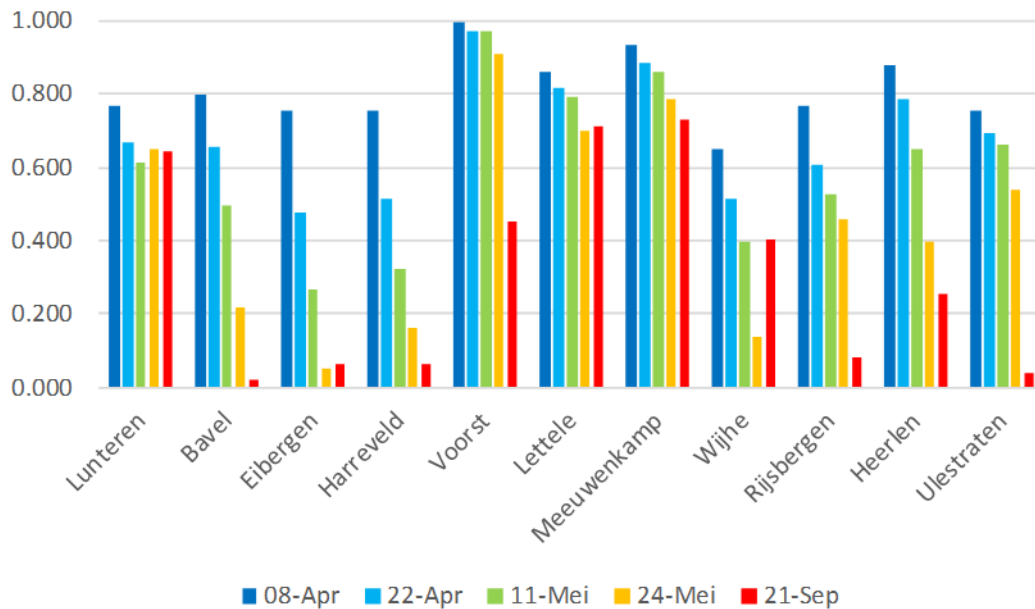
Figuur 93. Fractie beschikbaar bodemvocht voor de elf meetlocaties op vijf momenten in 2020.
