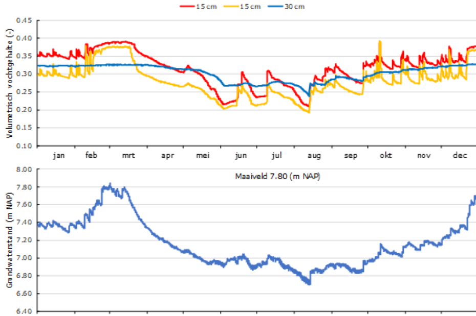
Figuur 94. Gemeten bodemvochtgehalte en grondwaterstand in het jaar 2020 op locatie Lettele. De bodemvochtmetingen op 30 cm diepte zijn betrouwbaar voor slechts één sensor.
