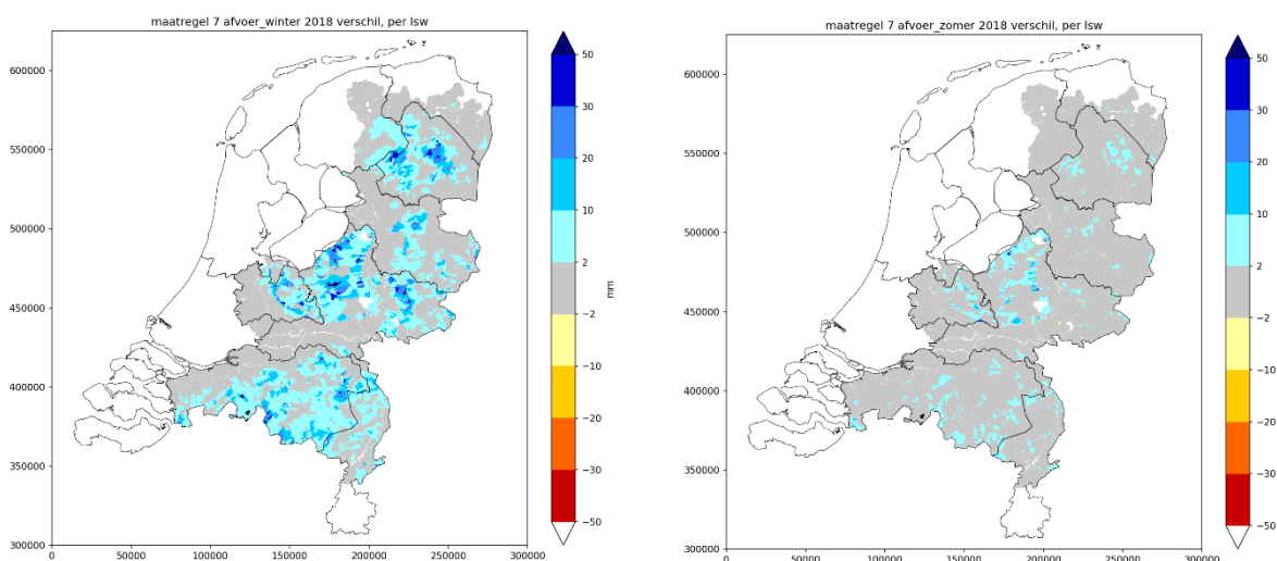
Figuur 72. Effect op de gebiedseigen afvoer door omvorming naaldbos naar heide, in de winter (links) en de zomer (rechts) van 2018.
