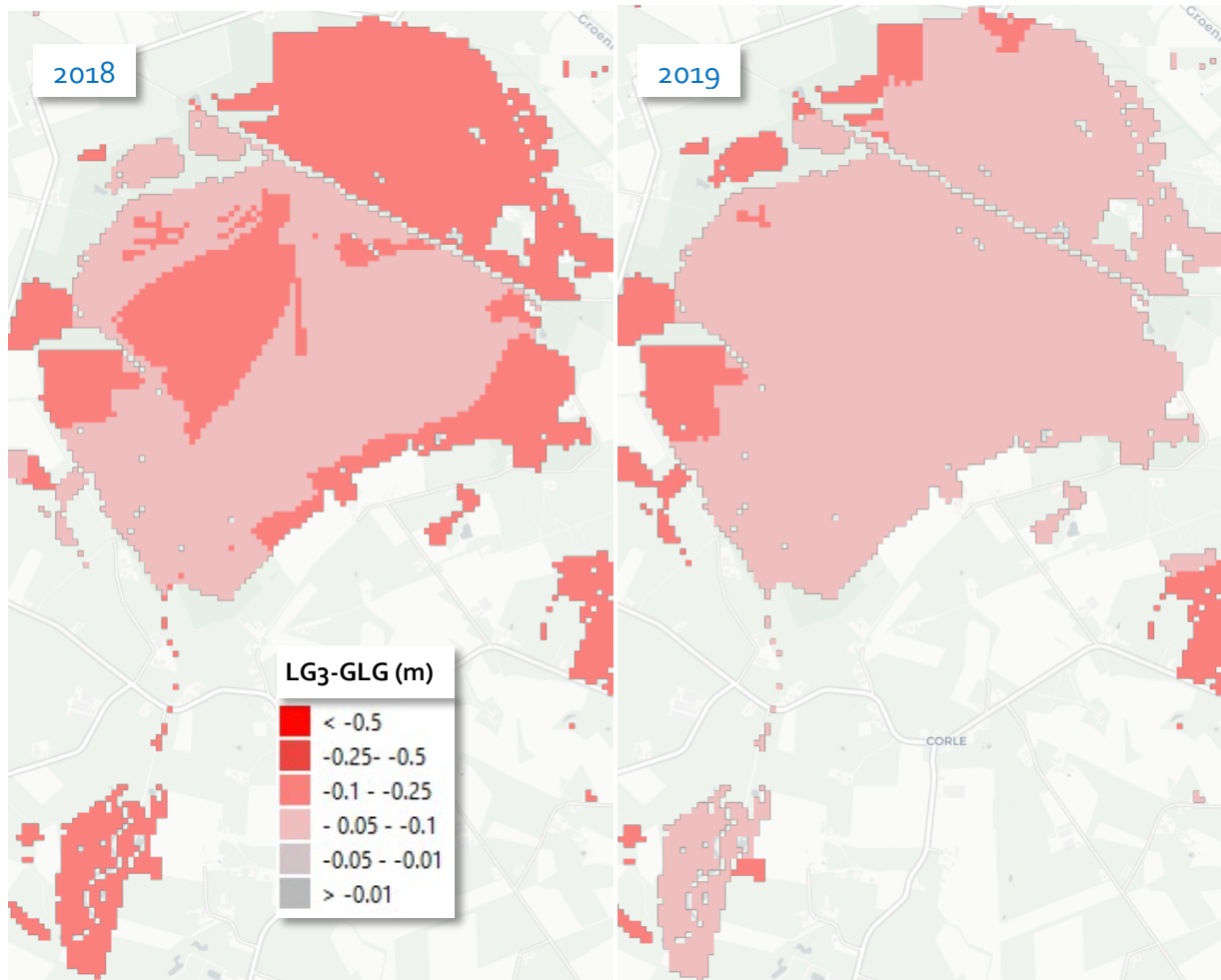
Figuur 22. Uitzakken laagste grondwaterstand in 2018 en 2019 (LG 3 -GLG) onder de grondwaterafhankelijke natuur van het Kornburgerveen.
