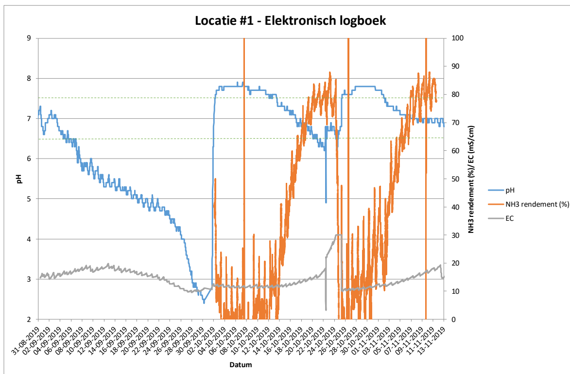
Figuur 4 Locatie #1 elektronisch logboek: De pH en EC van het waswater in de luchtwasser zoals geregistreerd in het elektronisch logboek. NH3 rendement is het berekende ammoniakverwijderingsrendement gemeten met de ammoniaksensoren. De gestippelde lijnen zijn de maximale (7,5) en minimale (6,5) pH-waarden die voorgeschreven staan voor een goed werkende biologische combi-wasser.
