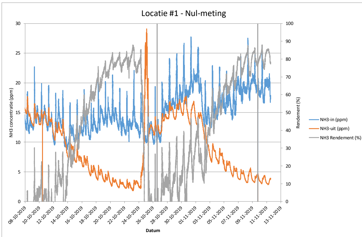
Figuur 3 Locatie #1 nulmeting: Overzicht van de gemeten ingaande (NH3-in) en uitgaande (NH3-uit) ammoniakconcentratie in ppm gemeten met de ammoniaksensoren samen met het berekende ammoniakverwijderingsrendement, meting vond plaats vanaf 8 oktober tot 11 november 2019.
