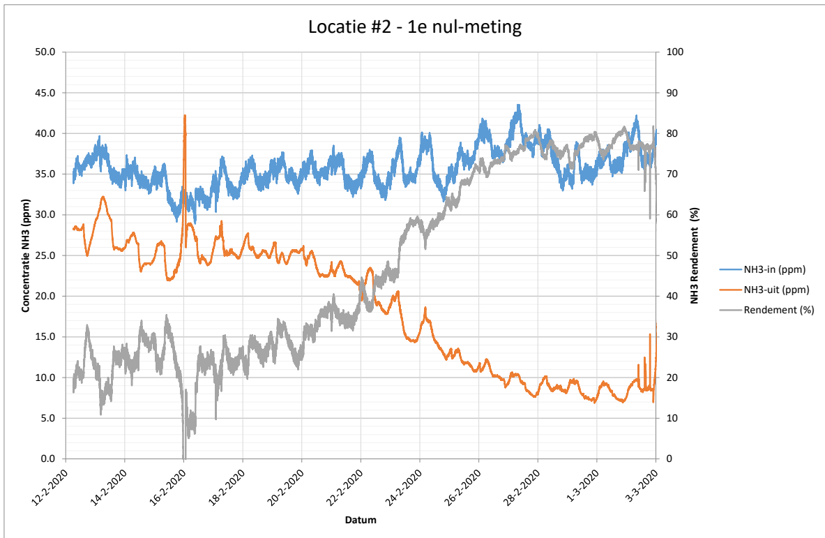
Figuur 7 Locatie #2 1 e nulmeting: Overzicht van de gemeten ingaande (NH 3 -in) en uitgaande (NH 3 -uit) ammoniak concentratie in ppm gemeten met de ammoniaksensoren samen met het berekende ammoniakverwijderingsrendement, meting vond plaats vanaf 12 februari tot 3 maart 2020.
