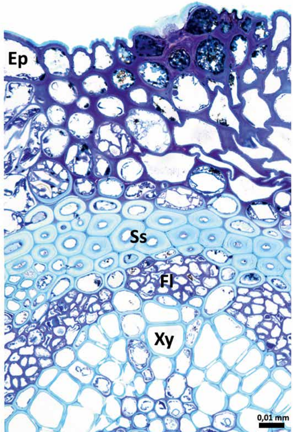
Figuur 2. (links) Dwarse doorsnede van een beukenblad met illustratie van de bladstructuren die mogelijk betrokken zijn bij bladwateropname. Een detailbeeld van desbetreffende structuren wordt in de cirkels weergegeven. Ep = epidermis, Pp = palisadeparenchym. Voor een uitgebreide anatomische beschrijving zie https://onlinemicroscopy.ugent.be/fagusNL.htm .
