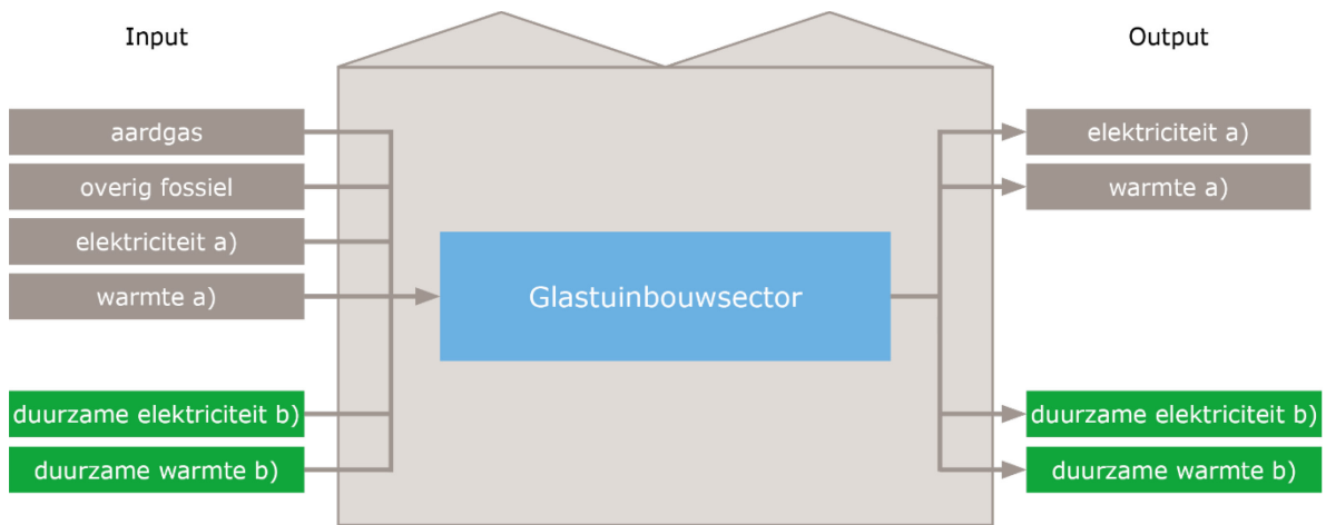
Figuur 2.4 Energie-input en -output glastuinbouw a) Fossiele bron; b) Hernieuwbare of duurzame bron.
