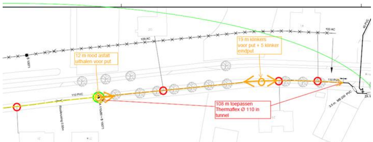
Figuur 3.1 Overzicht tracé in Berkel-Enschot met de ligging van de bestaande leiding. In oranje zijn de begin- en eindput aangegeven, in rood zijn de putten bij de aansluiting aangegeven. De tussenputten zijn niet aangegeven, voor 1 tussenput is het gat van de aansluiting gebruikt. De zomereiken zijn aangegeven met de grijze rondjes.
