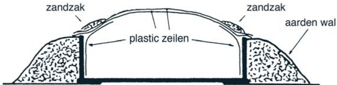
Figuur 5.1 Wijze van afdekken van een sleufsilos met uitsluitend folie
