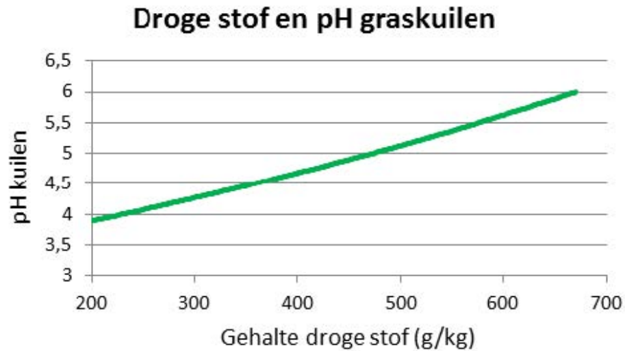
Figuur 5.2 Grenswaarden zuurgraad voor een goed geslaagde kuil bij diverse drogestofgehalten
