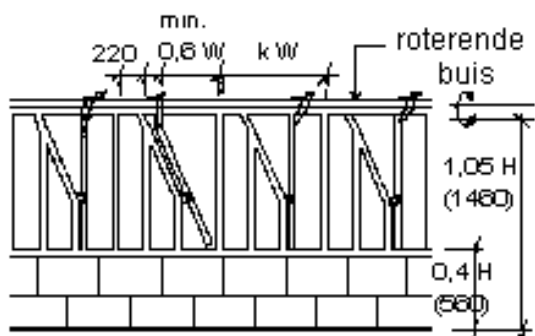
Figuur 30. Typische maatvoering van een zelfsluitend voederhek
