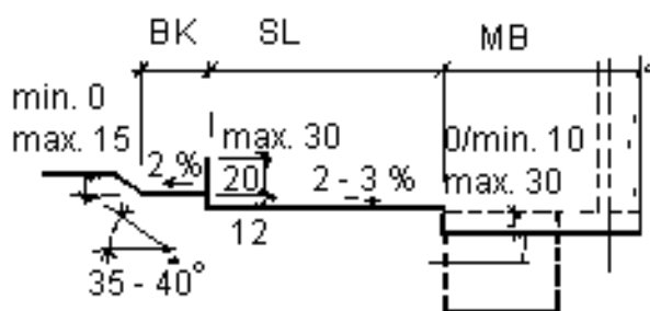
Figuur 23. Doorsnede van een korte stand
