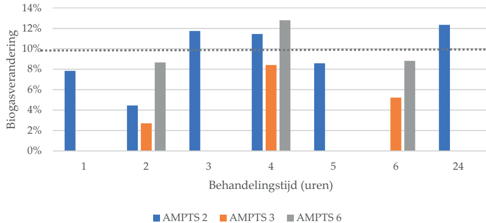
FIGUUR VI.12 RELATIEVE BIOGASTOENAME BIJ EEN BEHANDELING OP 55°C – AMPTS 2, 3, 6
