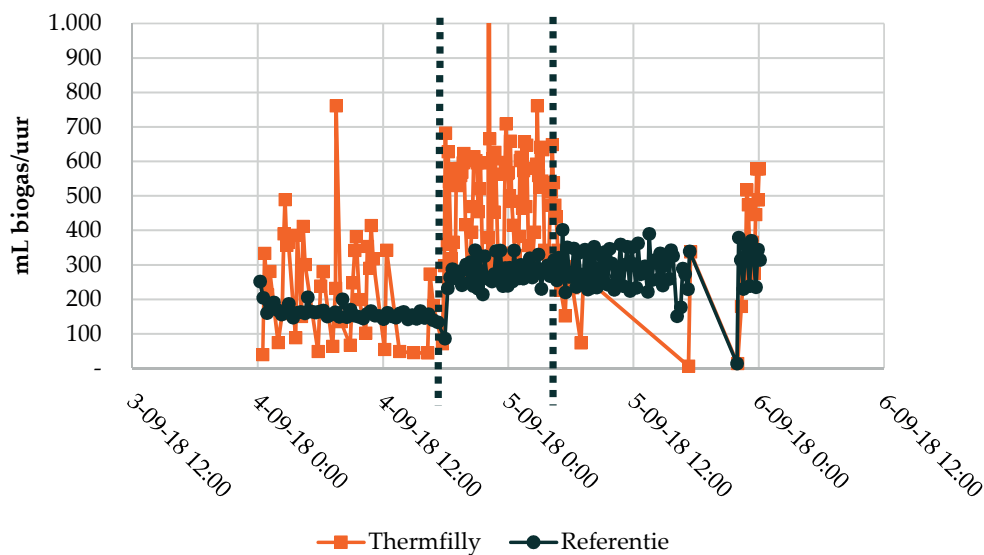
FIGUUR VI.21 PRODUCTIESNELHEID VAN DE REFERENTIE EN THERMFILLY REACTOREN VERGELEKEN. DE START VAN HET AANGEGEVEN GEBIED IS HET MOMENT DAT DE VOEDING VOOR BEIDE REACTOREN CONSTANT WAS. HET EINDE VAN HET AANGEGEVEN GEBIED GEEFT HET MOMENT AAN WAAROP DE THERMFILLY VOEDING OP RAAKTE
