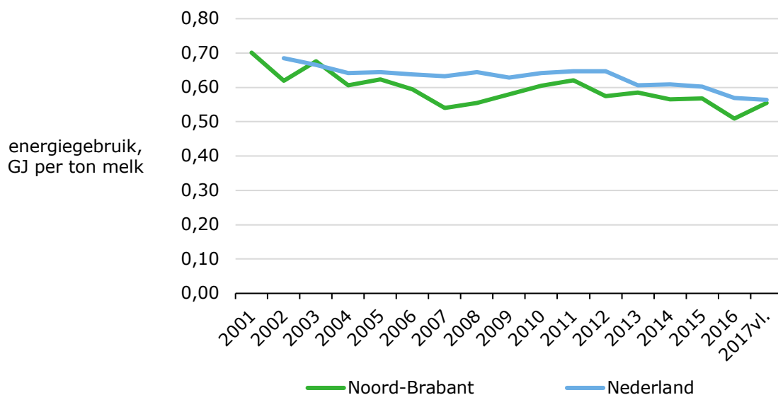
Figuur 14.3 Totale energiegebruik per ton melk op melkveebedrijven in Noord-Brabant en Nederland, 2001-2017vl.
