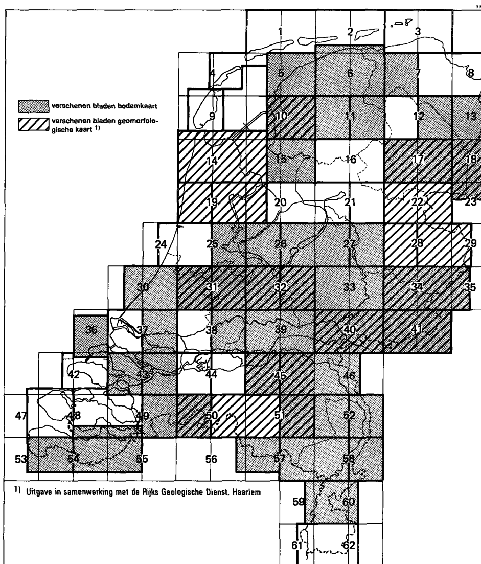
Afb. 2 Verschenen bladen van de Bodemkaart en van de Geomorfologische Kaart van Nederland, schaal 1:50 000, per 1-1-1984
