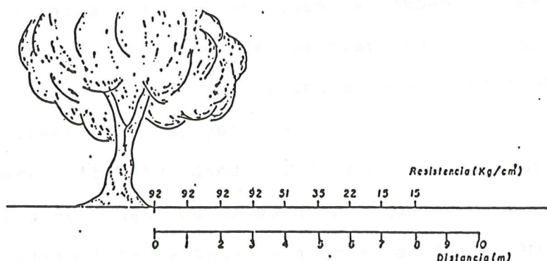
Figuur 1. Distributie van de penetrati weerstand in de bovengrond door sterke vertrapping van vee.
