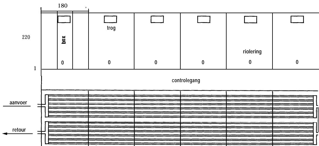
Figuur 1: Plattegrond van een kraamafdeling met volledig rooster (voorzien van een biggenest van 0,6 m 2 ) en R&R-mestkoelsysteem
