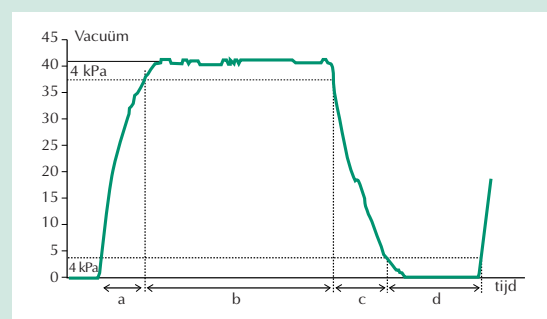
Figuur 1 Pulsatiekarakteristiek
