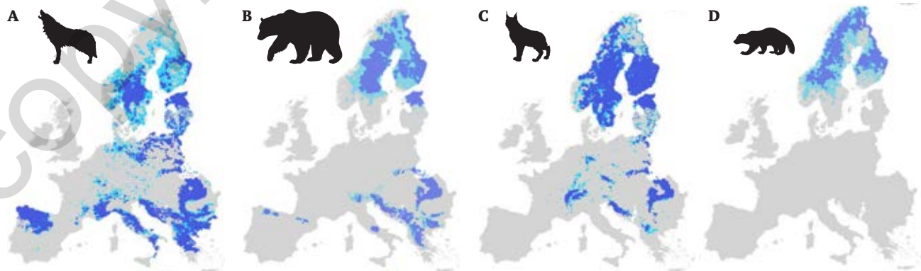
Geografische verspreiding van (A) de grijze wolf ( Canis lupus ), (B) de bruine beer ( Ursus arctos ), (C) de Euraziatische lynx ( Lynx lynx ) en (D) de veelvraat ( Gulo gulo ), de grootste marterachtige. De kaarten tonen de gebieden van permanente aanwezigheid (donkerblauw) en onregelmatige aanwezigheid (lichtblauw) in de periode 2012-2016. (Bron: Studie Europees Parlement – PE617.488)
