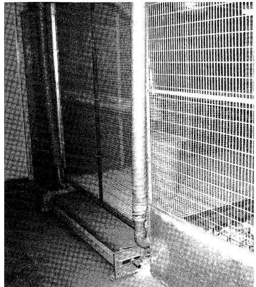
Opstelling van de gedeeltelijk (25procent) roostervloer in de kalkoenenstal. Onder het rooster-gedeelte zijn mestbanden en beluchtungs pijpen aangebracht.
