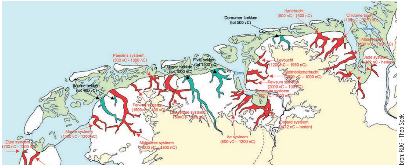
Afbeelding 2: Overzicht van het slenkensysteem langs de Duits-Nederlandse waddenkust. Marnesysteem (1560 v. Chr. - 1300 n. Chr.) als onderdeel reeks van laagten en actieve geulsystemen in open verbinding met de zee.
