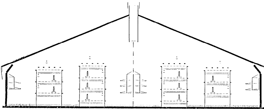
Figuur 2: het aangepaste etage-systeem met hellende roosters (op tekening niet te zien) en een vierde roostervloer (tekening: C. ter Beek, IMAG).
