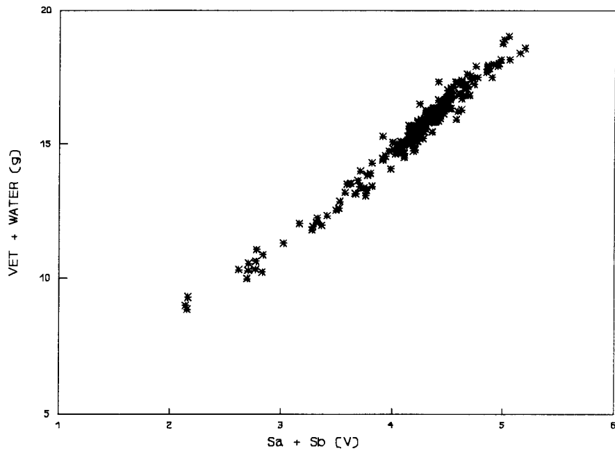
Afbeelding 1 - De som van de parameters Sa en Sb kan gebruikt worden om de som van het vet- en vochtgehalte te meten.
