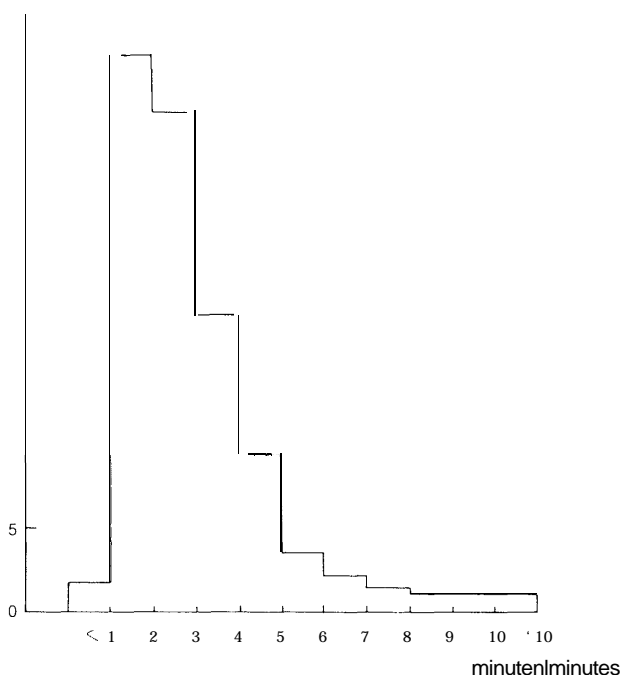
Figuur 3 Frequentieverdeling van de gemiddelde totale wisseltijden per 2 groepen van 8 koeien in 1984 t/m 1986
