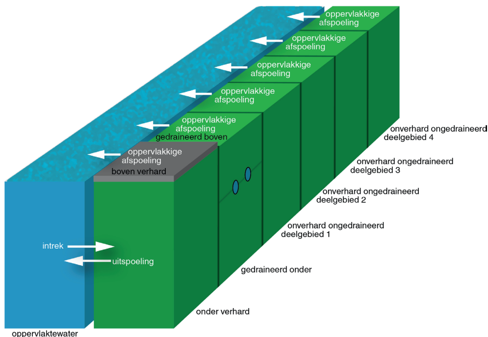
AFBEELDING 3.1 SCHEMATISCHE WEERGAVE VAN DE PERCEELBAKJES EN HET BAKJE OPPERVLAKTEWATER UIT DE WATERBALANS, EN DE WATERSTROMEN TUSSEN DE PERCEELBAKJES EN HET OPPERVLAKTEWATER (ZIE TABEL 3.1 VOOR EEN OVERZICHT WELKE WATERSTROMEN VOOR WELK PERCEELBAKJE VAN TOEPASSING ZIJN)
