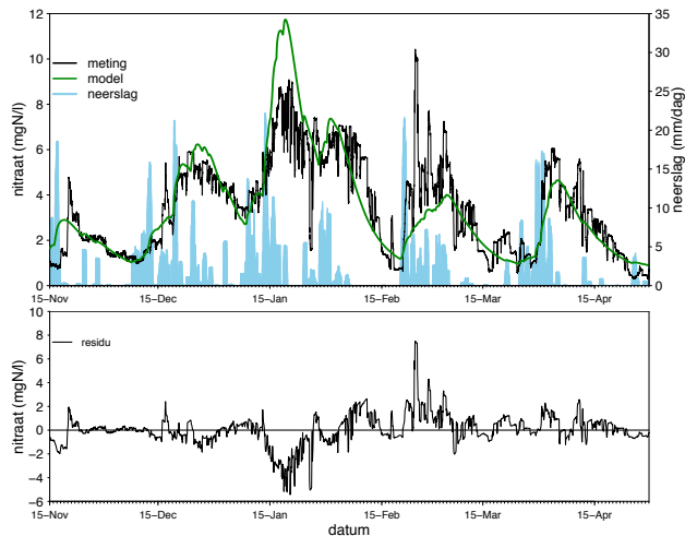
< Figuur 1 Hoogfrequente meetreeks voor nitraat, de neerslag (som van de voorafgaande 24 uur) en het tijdreeksmodel
