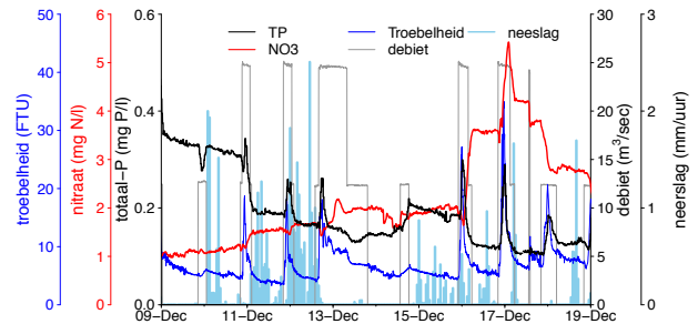
Figuur 2 Dynamiek in nitraat-, totaal-fosfor concentratie en zwevende stof (als troebelheid) na een natte periode op 10, 11 en 12 december samen met de neerslag en het pompegime
