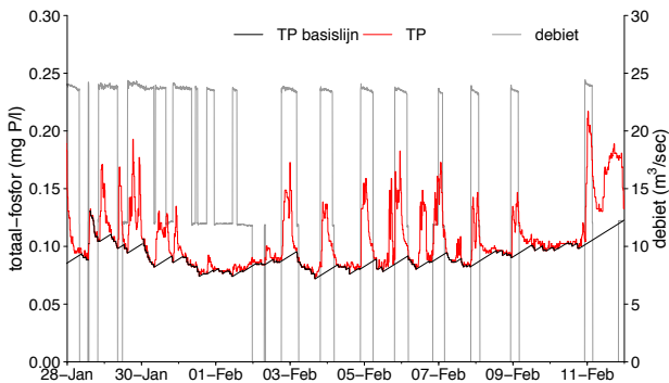
Figuur 3 Verandering van de TP-concentratie tijdens bemaling
