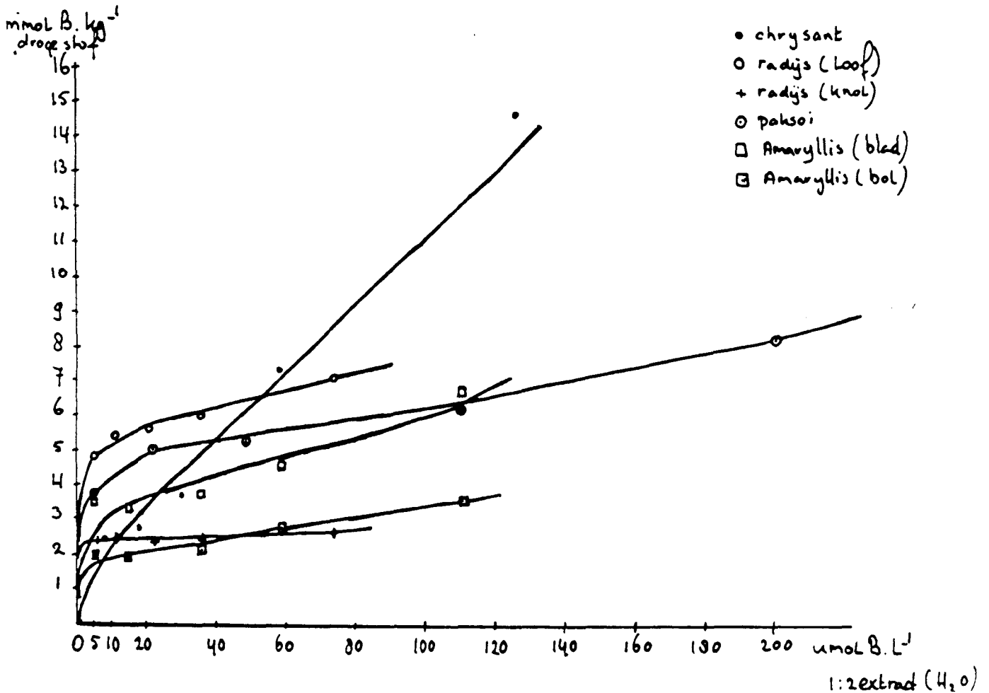
Figuur 5. Het verband tussen het boriumberhalte van de grond (1:2 volume extract \mu\text{mol/l} ) en het boriumberhalte van enkele gewassen ( \text{mmol/kg} droge stof).
