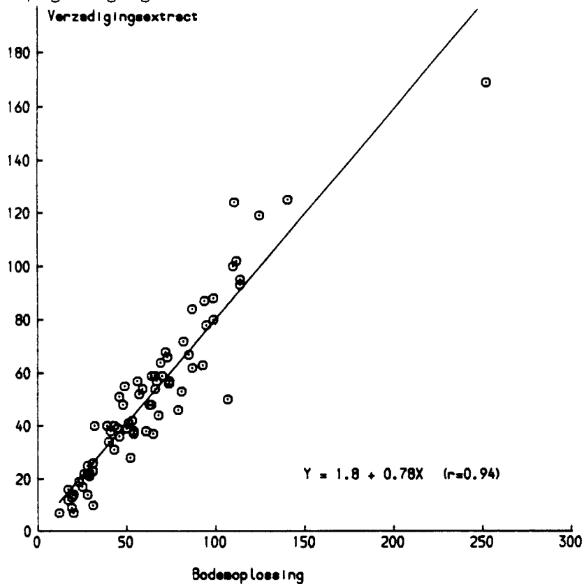
Fig. 1. De relatie tussen boriumgehalten in bodemoplossing en verzadigingsextract bij 75 kasgrondmonsters.
