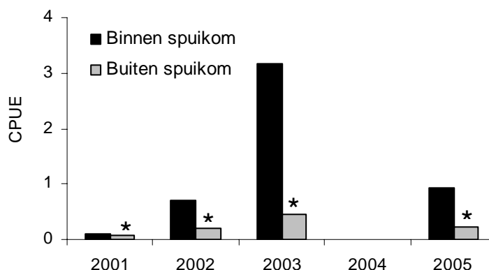
Figuur 5.23 Verskil in fintvangsten binnen en buiten de spui kom in het diadrome vissen programma in de periode 2001-2005 (ex 2004). Een * geeft aan als er met het keerwant gevist is (in 2001 is er aan de buitenzijde in het voorjaar zonder en in het najaar met keerwant gevist)
