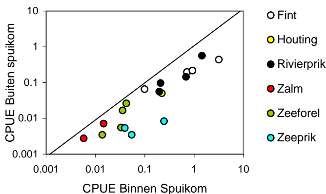
Figuur 7.2 Jaarlijkse vangsten in CPUE binnen en buiten de spuiikom. De lijn geeft aan wanneer de vangst binnen de spuiikom gelijk is aan die buiten de spuiikom. Ieder punt geeft 1 jaar weer.
