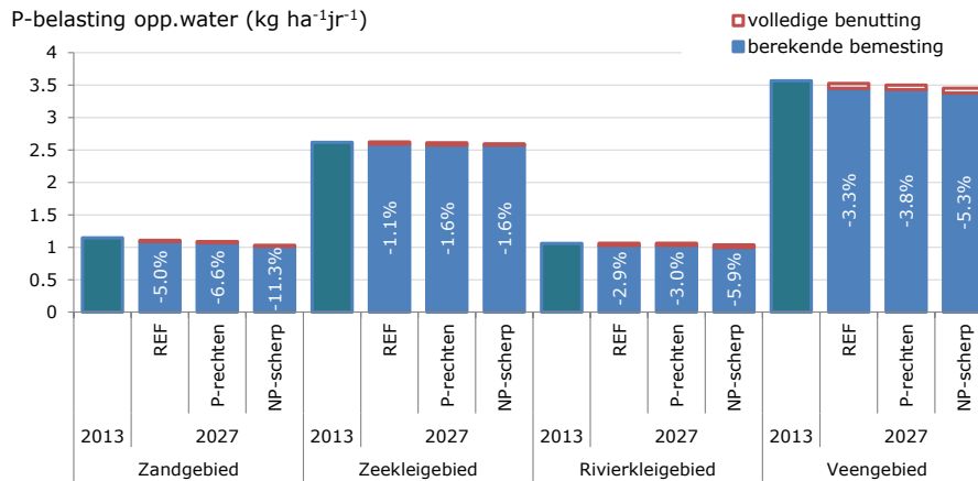
Figuur 25 P-belasting van het oppervlaktewater (kg ha -1 jr -1 ), gemiddeld voor alle landbouwgronden in het zandgebied, het zeekleigebied, het rivierkleigebied en het veengebied. De vermelde percentages geven de daling aan ten opzichte van de berekende P-belasting van het oppervlaktewater in 2013.
