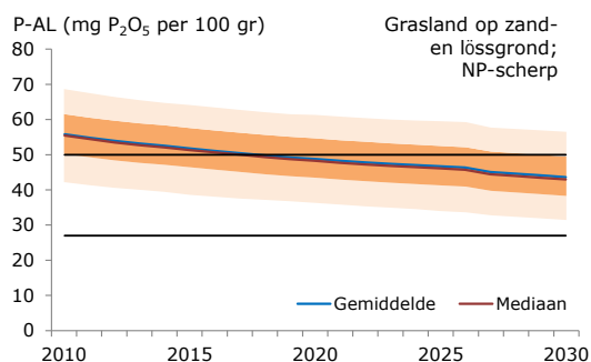
Figuur 69 Berekende ontwikkeling van de P-AL-waarde (mg P 2 O 5 per 100 gr) en bijbehorende bandbreedte van de ruimtelijke spreiding onder grasland op zand- en lössgrond (links) en onder grasland op kleigrond (rechts) bij berekende bemesting in het NP-scherpsceario. Horizontale lijnen duiden de grenzen aan tussen de klassen "laag", "neutraal" en "hoog".
