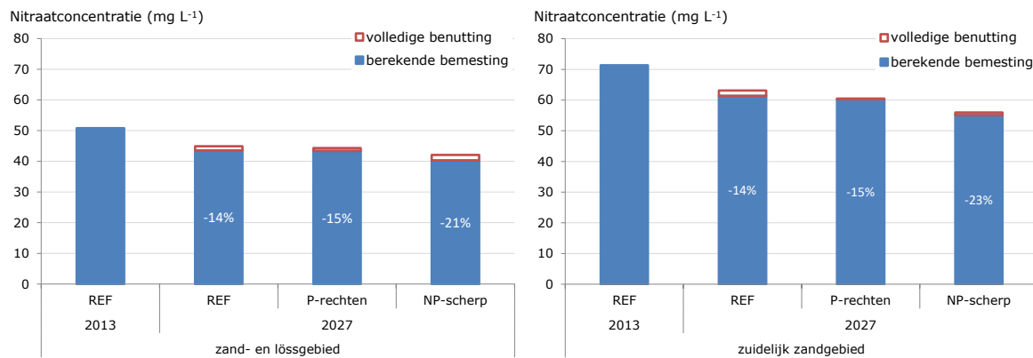
Figuur 16 Gemiddelde nitraatconcentraties ( \text{mg L}^{-1} ) in de bovenste meter van het grondwater, berekend voor het gehele zand- en lössgebied (links) en het zuidelijke zandgebied exclusief het lössgebied (rechts) waarbij gecorrigeerd is voor effecten van weersvariatie. De vermelde percentages geven de daling aan ten opzichte van de berekende nitraatconcentraties in 2013.
