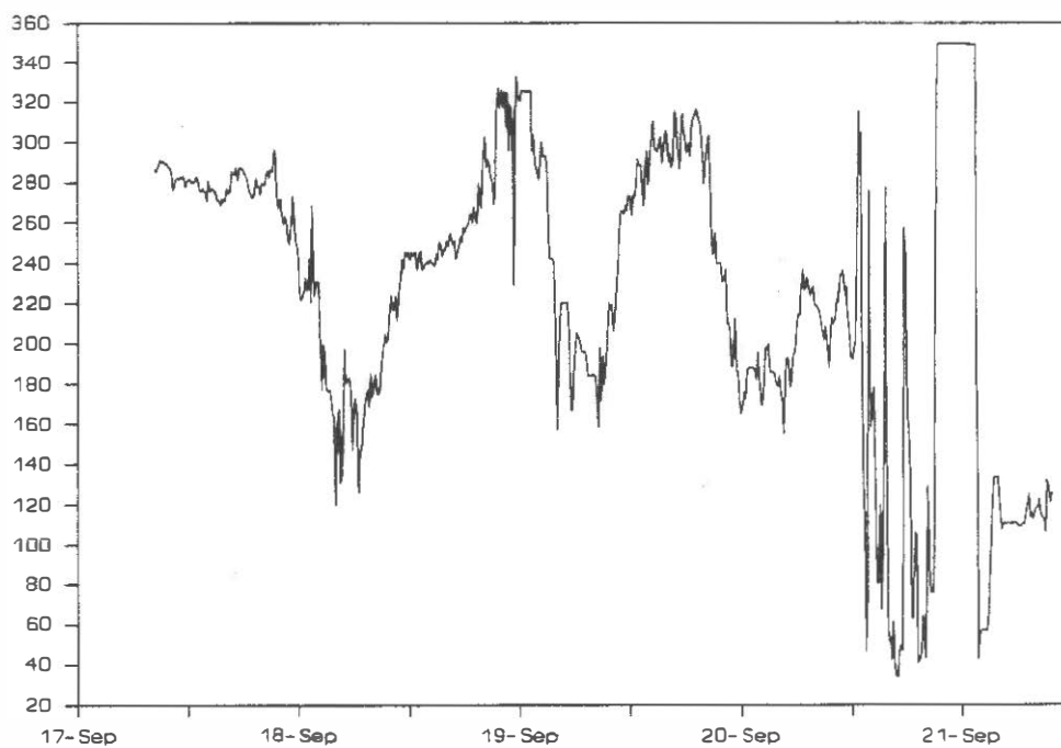
Figuur 7. Windrichting.
