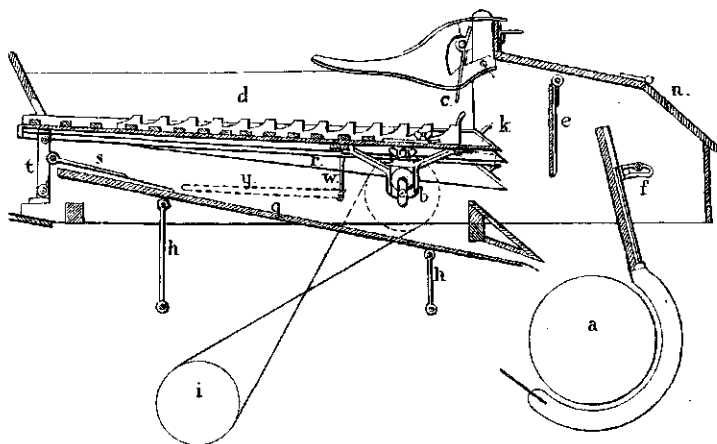
Fig. 90. Wilder's zelfvoeder voor eene stoomdorschmachine: a , dorschcilinder; b , krukassen; c , heen- en weergaande tanden ( s ); d , schudborden (5) van tegenhoudende tanden (ratched teeth), k , voorzien; e , loshangend bord; f , vast bord; n , deur, die geopend kan worden om het koren in te steken als de zelfvoeder defect is ( f wordt in dit geval teruggeslagen); r , veiligheidsbord; g , schudbord, in beweging gebracht door den drijfstang s en ondersteund door de stangen h ; w , staaf met hefboom j ; i , schijf met riem zonder eind waardoor de krukas b hare beweging ontvangt.
