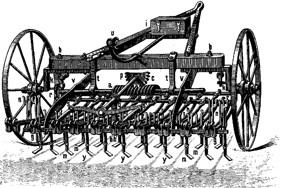
Fig. 40. Schoffelmachine volgens Taylor, passende bij de zaaimachine, Fig. 10: hh' , hefboomen; m , mesjes; y , op rijen gezaaid graan; g , gewichten; i , kistje tot berging van schroefdraaiers, enz.; ss' , hefboom om te sturen; pc , halftandrad; a , staaf met schroef zonder eind; tt , ijzers met oogen; vv , ijzers voor het opbeuren der hefboomen; vv , staven waaraan de hefboomen bevestigd zijn; kk , geknikte as der wielen; u , haak om de hefboom ss in te slaan bij het uit 't werk zetten; nn , vorken om enkele hefboomen buiten 't werk te zetten; g , ijzeren staaf, waaraan de dwarsstaaf gg is bevestigd; bb , schroefhouten.
