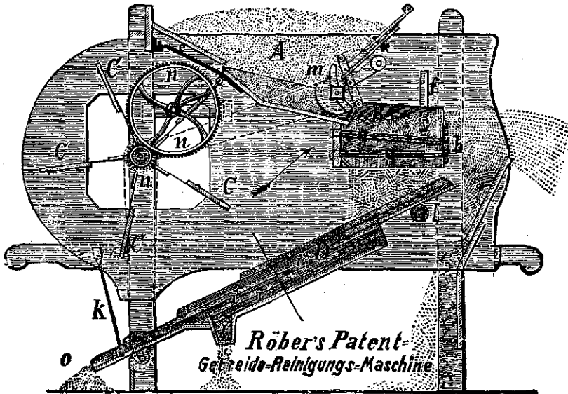
Fig. 103. Wanmolen „Ideal” van Gebr. Röber te Wutha, Thüringen.
