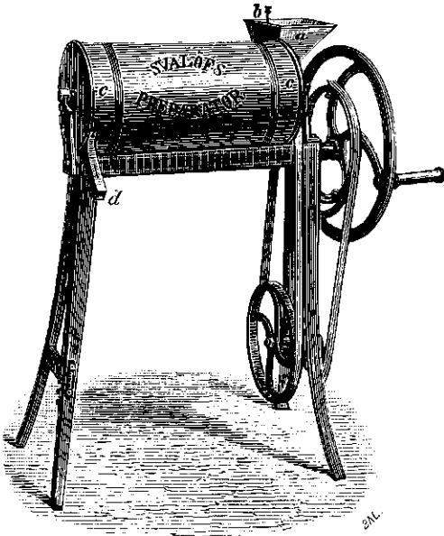
Fig. 1. Zweedsche krasmachine voor klaarzaad.
