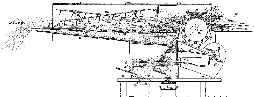
Fig. 87. Hekeldorschmaschine met schoontoestel van Stout te Tiel, op \frac{1}{30} der ware grootte: a dorscilinder; t , tanden of stiften (kiezen); p , blok met tanden; g , ongedorscht graan; n , strooschudders; o , harken voor het opschudden van 't stroo; v , reepen leer, aan den onderkant vrij hangend, voor het tegenhouden der korrels; r , krukassen; b , stroozeef; c , schudbord; z , eerste en z' , tweede zaadzeef; s en s' , drijfstangen, verbonden aan excentrieken om de as van den waaier d ; q , gootje voor het opvangen van ongedorschte aren, die uit t met den jakobsladder e i weder naar de dorschtrommel worden gevoerd; k , gootje voor den uitloop van 't zaad; m , maat om dit op te vangen.
