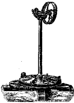
Fig. 79. Zuilrosmolen met kegebraderen van H. Lanz te Mannheim.
