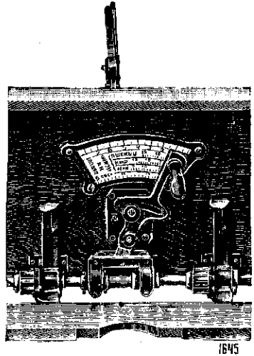
Fig. 26. Schaal met hefboom voor het stellen der schepraderen van Eckert's breedzaaimachine en voor het aanwijzen van de juiste hoeveelheid te zaaien zaai-zaad.
