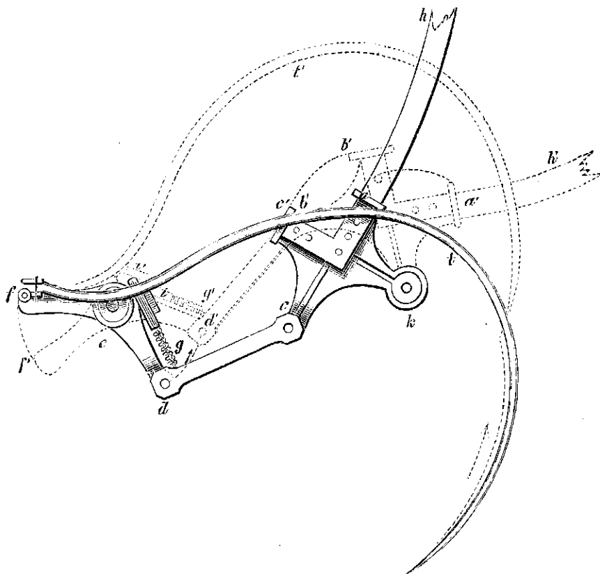
Fig. 56. Doorsnede van Ransomes' hooihark, zonder zitplaats, langs den hefboom, om te doen zien, hoe de tanden opgebeurd worden: abcdef , kniehefboom; k en e zijn vaste punten. De stippellijnen stellen den stand der tanden en van den hefboom voor, wanneer h naar beneden wordt gedrukt; de geaccentueerde letters wijzen de verschillende deelen in dezen stand aan; t en t' , staaf voor het opheffen der tanden; g en g' , veer.
