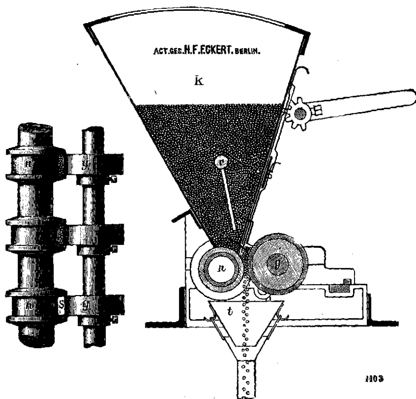
Fig. 20. De zaadkast k van de vorige figuur: daaraan rechts de schuif om den toevoer van het zaad s te regelen. De zaadkast wordt van onderen gesloten door de nokkenwals r , waartegenover de schijvenwals y geplaatst is. Gedeelten van beide walsen zijn in de figuur links van bovenop gezien voorgesteld; t , trechter; r , roer­toestel.
