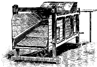
Fig. 85. Dorschmachine van H. Lanz, met terrasvormig geplaatste zeven en harkvormige strooschudders.
