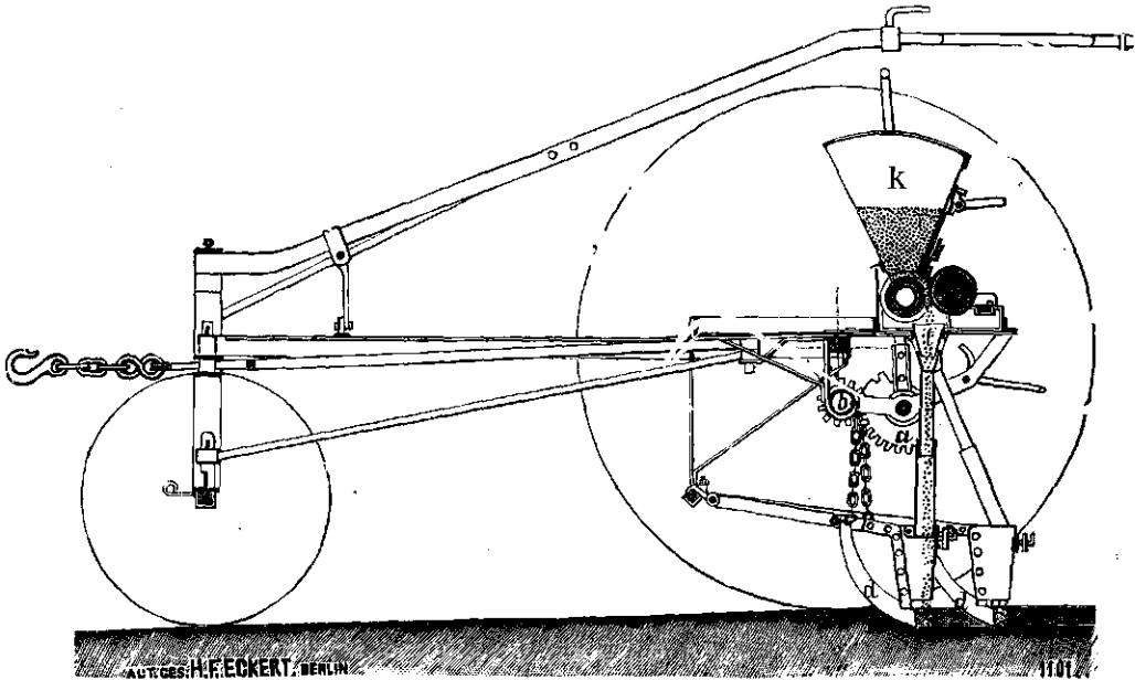
Fig. 19. Zaaimachine van Eckert, agent Ch. R. Kouveld, Amsterdam, lengte-door-snedede: k , zaadbak; a , gedeelte van een tandrad, dat in het tandrad b grijpt op de as bevestigd, waaraan de kettingen voor het opheffen der hefboomen; d , voentrekkers.
