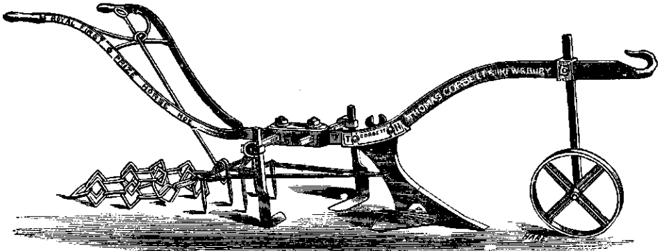
Fig. 35. Corbett's aanaardploeg als paardenbak of schoffelploeg ingericht.
