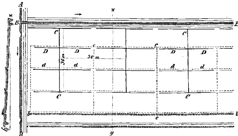
Fig. 255. Plan eener bevloeiing volgens eene richting ( Hangbau ): A, A , hoofd-aanvoerkanaal; B, B , dwarskanaal voor aanvoer van water; C, C , verdeelingskanalen; D, D , bevoeiingsgreppels; b, b , dwarskanaal voor den afvoer van water; c, c , verzamelkanalen; d, d , verzamelgreppels; x, y , dwarsprofiel.
