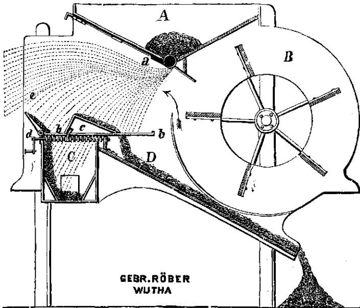
Fig. 101. Wanmolen voor het sorteeren van granen van Gebr. Röber te Wutha, Thüringen, in doorsnede.
