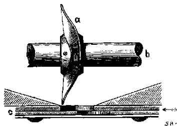
Fig. 24. As met schoepschijf van Eckert's breedzaaimachine.
