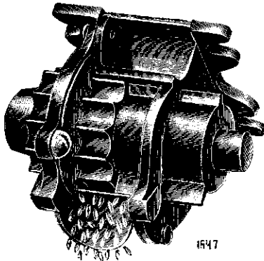
Fig. 25. As met scheprad van Eckert's breedzaaimachine.
