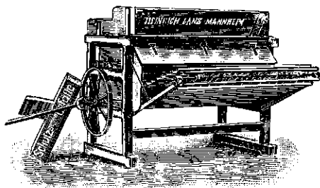
Fig. 86. Dorschmachine met slaglijsten, trommel en rondlopende strooschudders van H. Lanz te Mannheim.
