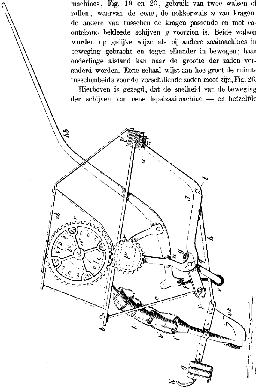
Fig. 10. Doorsnede van een vereenvoudigde zaaimachine, in het noorden van Groningen in gebruik, om te doen zien de wijze waarop de vorentrekkers worden opgeheven en de machine terzelfder tijd uit het werk wordt gezet. lkk 1 , hefboom van den vorentrekker vt ; g , gewichten; zb , zaadbak; l 1 l 2 , vaste trechters; l , in elkaar schuifbare trechters; k 1 , kettingen; r 1 , wielrad; r , lepelrad; a 1 , as van het lepelrad; l , lepels; p 1 , wielas; p , andere vaste as der machine; d , gebogen ijzeren staaf; hb , hefboom, met daaraan bevestigde stang f , dwarsstaaf e en hefboom q ; ab , hefboom voor het opheuren van den zaadbak; c , staaf.
