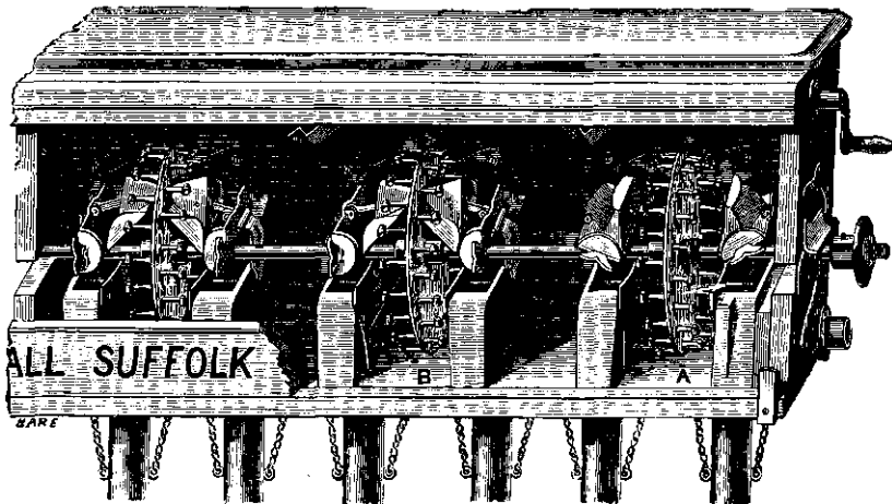
Fig. 6. Gedeelte der zaadkast van Smyth's zaaimachine; bij A zijn de trechters terug geslagen of in den stand om de as te kunnen nitnemen; bij B in den stand om te zaaien.
