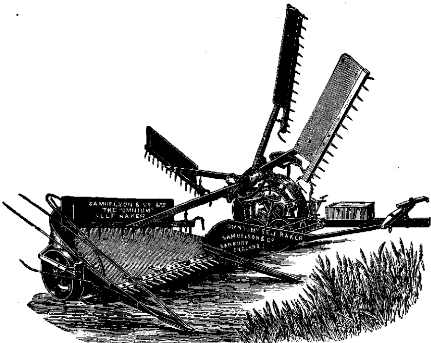
Fig. 49. Zelf-schoovenvormende graanmaaiër van Samuelson & Co. te Banbury.
