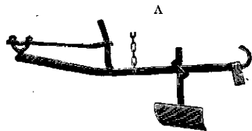
Fig. 31. A. Een der hefboomen van Sack's schoffelmachine, voorzien van een strijkbordereu voor het bedekken van gelegde aardappelereu; B, idem met vorentrekker en marqueurradereu, zie Fig. 29, voorzien.
