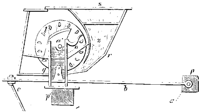
Fig. 5. Doorsnede van den zaadbak eener zaaimachine, om de verdeeling van het zaad te doen zien. De gestippelde lijnen in den zaadbak S wijzen ongeveer den loop van het zaad aan. a' , as der lepelschijven; qo , opsluitijzer; p , as der machine; ab , hefboom, draaibaar bij a ; c , staaf.
