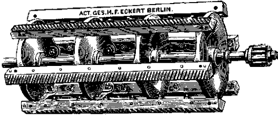
Fig. 66. Dorschtrommel met slaglijsten van Eckert's dorschmaschine.
