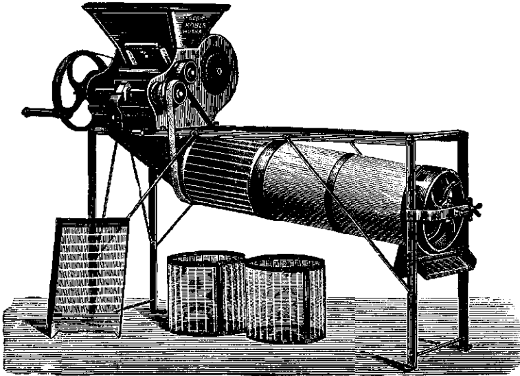
Fig. 106. Mayer's eenvoudige trieur met schud- en cilinderzeeven, van Gebr. Röber te Wutha (Thüringen).
