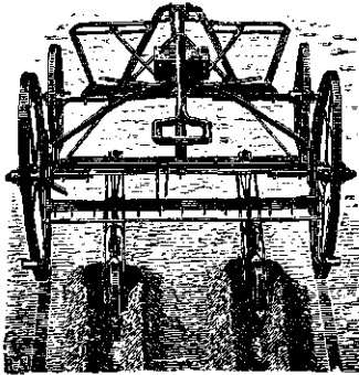
Fig. 29. Het 1 1/4 M. breed zaaiwerktuig van Sack, ingericht als aardappelvorentrekker met marqueurradereu (Fig. 31, B) voor 2 rijen.
