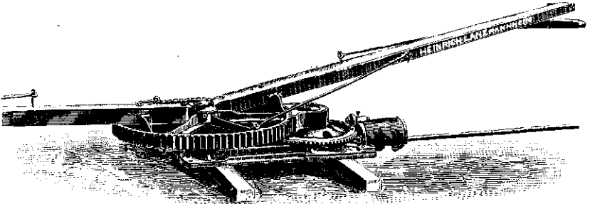
Fig. 72. Rosmolen van H. Lanz te Mannheim; waar de tandraden in elkander grijpen zijn deze overdekt, zoomede de plaats waar de twee koppelstangen samenkomen.
