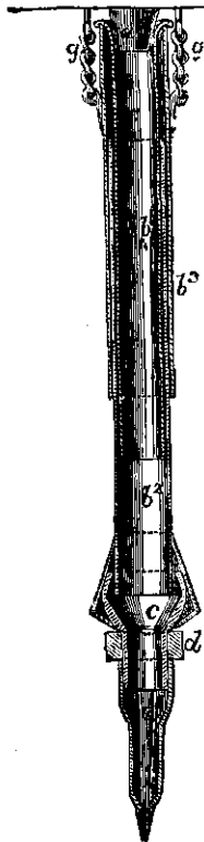
Fig. 7. Telescopische trechters van Sinyth's zaaimachine.
