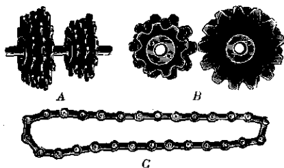
Fig. 18. Trapvormige tandraderen: A , op zij; B , van voren gezien; C , ketting zonder eind in Sack's zaaimachine, klasse III en IV.
