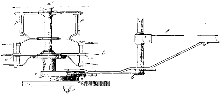
Fig. 53. Doorsnede der rechtsche helft van een hooischudder (van Howard): a, as van de wielen waarop de machine rust; a', as van den haspel; c en c', overdekte tandraderen, waardoor de beweging der wielen op den haspel wordt overgebracht; b, stang, waarmede de machine gesteld kan worden; t, tanden, die bij p teruggeslagen en daarom onzichtbaar zijn; v, veeren; l, limoen.
