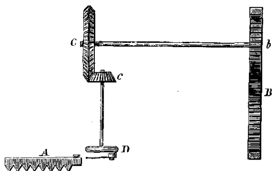
Fig. 45. Schematische voorstelling van de overbrenging der beweging in eene maaimachine: B, tandrad in een der wielen, waarin het kleiner tandrad b grijpt; C, c, kegelraden; D, excentrische schijf of krukas; A, mes.
