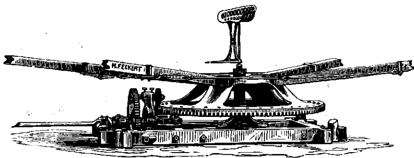
Fig. 70. Klokvormige rosmolen met vaste tusschenbeweging van Eckert te Berlijn. Agent Ch. R. Kouveldt te Amsterdam.
