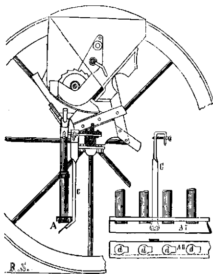
Fig. 22. Inrichting voor Sack's zaaimachine, klasse II, III en IV en ook voor klasse I met hooge wielen van 1\frac{1}{4} M. breedte voor het breedwerpig zaaien van vlas- en klaverzaad: A, op zij; AI, van voren; AII, van boven gezien. C, staven om het toestel aan de machine te hangen. Aan het schuin aflopende benedeneinde daarvan is een hoekig gebogen plaat bevestigd, waarvan het horizontaal gedeelte van openingen d is voorzien om de zaaihuizen door te laten en het hellende gedeelte daaronder geplaatst om het uit de buizen vallende zaad te doen afloopen.
