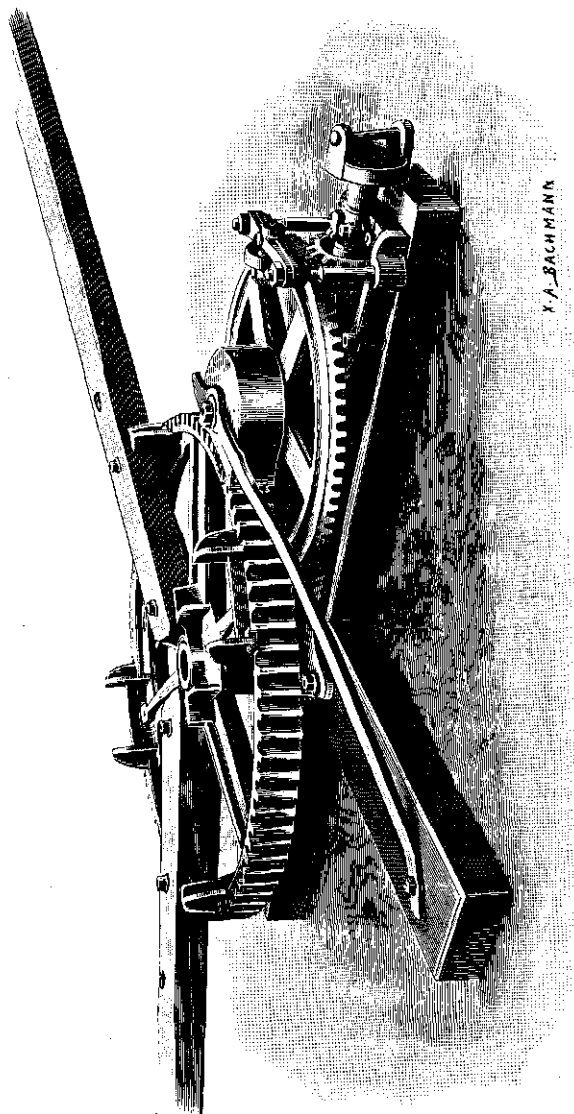
Fig. 69. Rosmolen van Joh. Rauschenbach te Schafhausen en Frankfurt a/M. met palrad en koppelstang; het eene kamrad is overdekt.
