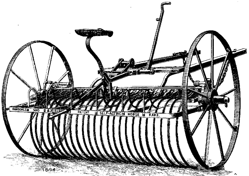
Fig. 55. Ransomes zelfwerkende hooihark.
