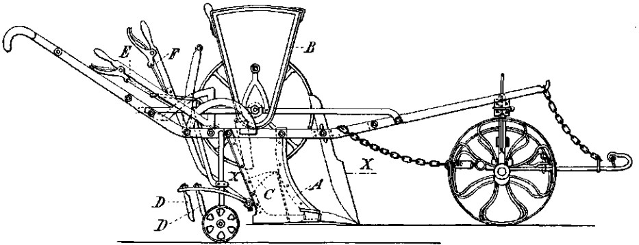
Fig. 252a. Ondergrondbemestingsploeg van P. Gross te Hohenheim, naar die van Fuchs eenigszins gewijzigd en bij het Breiner proefstation in gebruik voor het bemesten van veengronden, vooral met mergel en kalk, in lengte-doorsnede.
