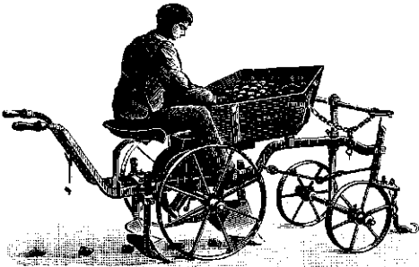
Fig. 28. Aardappelpootmachine van A. Bajac te Liancourt (Oise). Het stel kan ook als paardehak, als aanaardploeg en als aardappelrooier worden ingericht.
