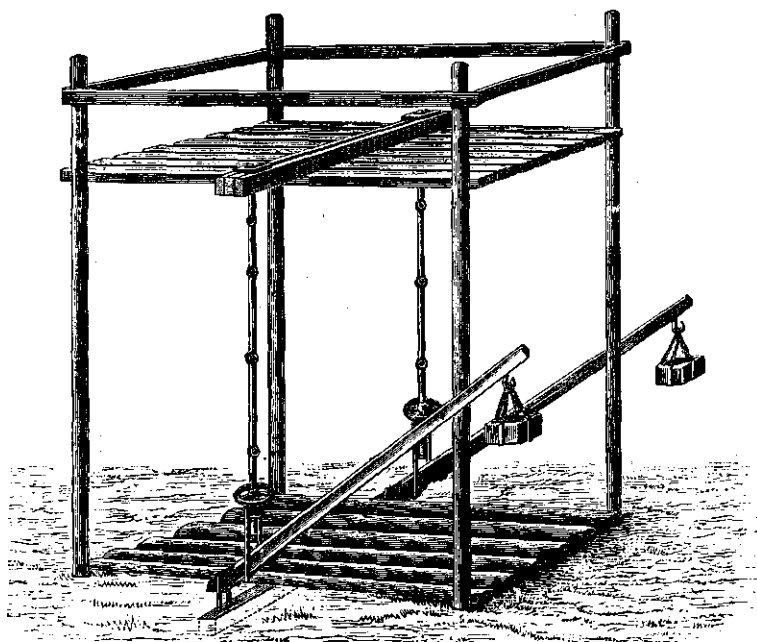
Fig. 61. Blunt's groenvoederpers, agent G. Stout te Tiel.
