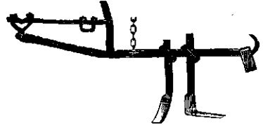
Fig. 37. Een der hefboomen van Sack's schoffelmachine op zij gezien met een hakmes E en een korstmes K , Fig. 39.
