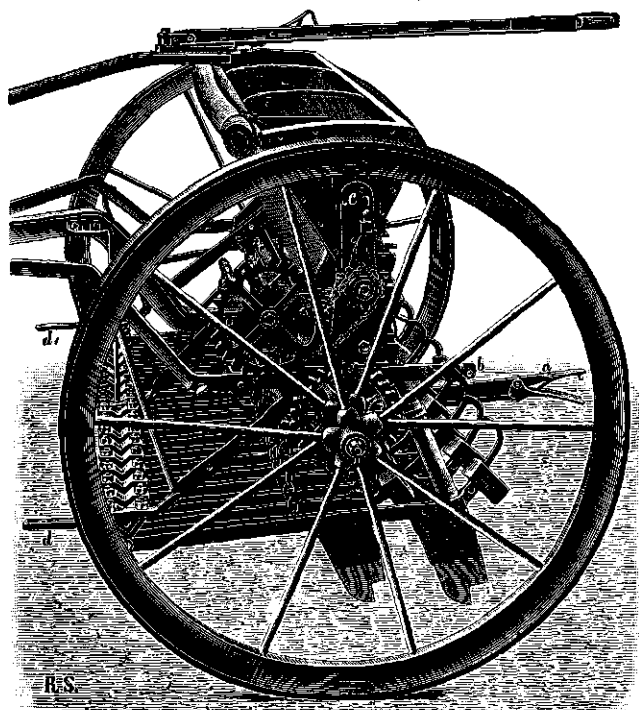
Fig. 17. Sack's zaaimachine, klasse III, uit het werk gezet: a , hefboom; d , drager voor de schraapijzers om de raderen schoon te houden, opdat geen modder in den zaadhak valt; c , schroeven om de plaat waarop de zaaias rust te bevestigen; dd' , dragers voor het toestel, Fig. 22, om klaverzaad te zaaien.
