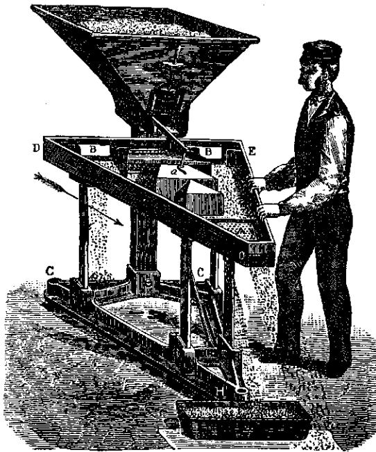
Fig. 110. Sorteertafel of Cribleur van Josse: T, bak voor het laten toevloeden van 't graan; DEO, sorteertafel; B, openingen voor het doorlaten van lichte voorwerpen; a, driehoekige lichamen; A, zeef; CCH, grondraam, bij CC op vaste pooten rustende, bij H op een stelschroef.
