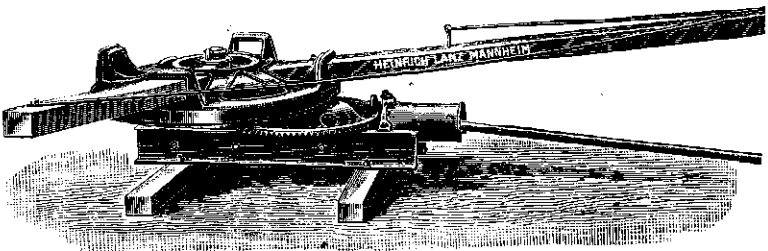
Fig. 73. Veiligheidsrosmolen van H. Lanz te Mannheim.
