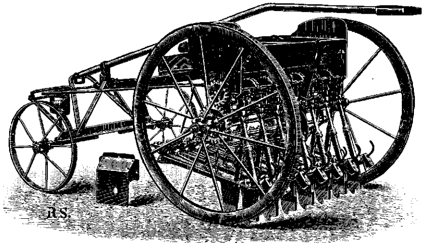
Fig. 12. Sack's zaaimachine, klasse I met hooge wielen en schokbreker; de kast voor het beschutten der tandraden is afgenomen.
