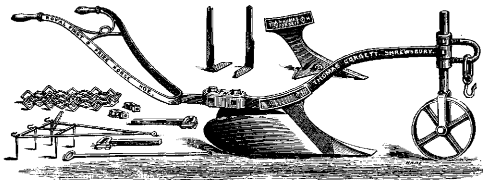
Fig. 34. Aanaardploeg met daarbij passende deelen om hem als paardehak in te richten van Thomas Corbett te Shrewsbury.
