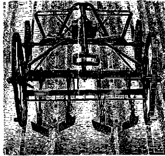
Fig. 30. Dezelfde machine als Fig. 29 met strijkbordereu om de gelegde aardappelereu met grond te bedekken. Zie de inrichting op zij gezien in Fig. 31, A.
