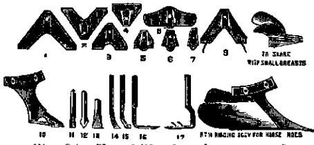
Fig. 36. Verschillende scharen enz. behorende bij Corbett's schoffelmachine.
