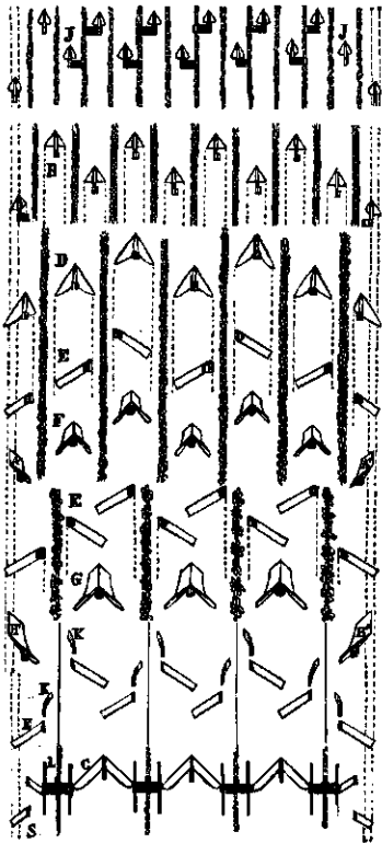
Fig. 39. Verschillende scharen en messen van Sack's schoffelmachine: J, tweesnijdend bladvormige schaar van 7 cM. snijbreedte; B, idem, van 8—12 cM. snijbreedte; C, idem, van 23—40 cM. snijbreedte; D, idem, van 13—22 cM. snijbreedte; E, éézijdig schoffelmess met afgeronde hoeken van 14—20 cM. snijbreedte; F, aanaarder voor 20—36 cM. rijenwijdte; G, idem, voor 37—50 cM. rijenwijdte; K, korstmess; H, schaarvormig mes om aan te aarden.
