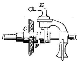
Fig. 47. Maaimachine uit het werk gezet.
