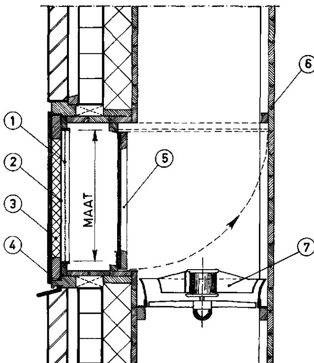
AFB. 21. Doorsnede over luchtinvoeropening met luik.
