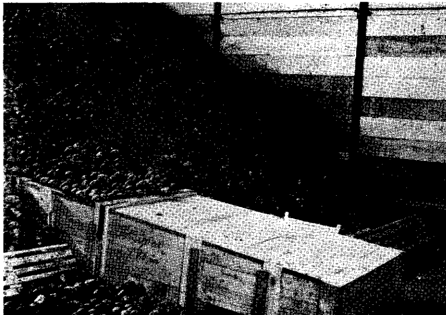
Afb. 17. Wegneembaar bovengronds houten luchtverdeelsysteem. De aardappelen liggen hier opgeslagen tussen z.g. montagewanden. Het luchtverdeelsysteem en de wanden zijn wegneembaar. De wanden bestaan uit op zichzelf staande ijzeren steunen, die onderling zijn verbonden door trekstaven. De steunen zijn gemaakt van dubbel U-profiel. In het U-profiel worden de planken geschoven. Dergelijke bewaar ruimten worden veelal gebruikt in bestaande gebouwen voor tijdelijke bewaring van aardappelen gedurende de herfst.
