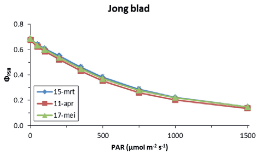
Figuur 4 Lichtrespons van de elektronentransport-efficiency door fotosysteem II ( \Phi_{\text{PSII}} ) van jonge bladeren op drie tijdstippen (gemiddelde \pm standaardfout, n = 5 ).
